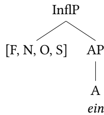
Figure 5.8: Structure of adjectival ein
