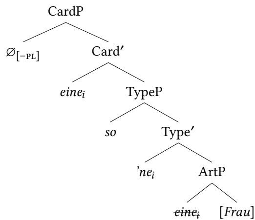
Figure 8.1: EINE so'ne Frau \emptyset_{[-PL]} +a so.a woman.FEM 'one such woman'
