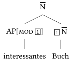
Abbildung 5.6: Kopf-Adjunkt-Struktur (Selektion)
