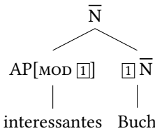
Abbildung 3.6: Kopf-Adjunkt-Struktur (Selektion)
