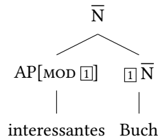
Abbildung 3.6: Kopf-Adjunkt-Struktur (Selektion)
