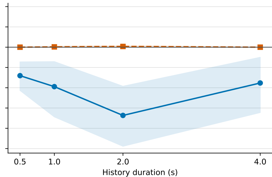
Qwen3-ASR
