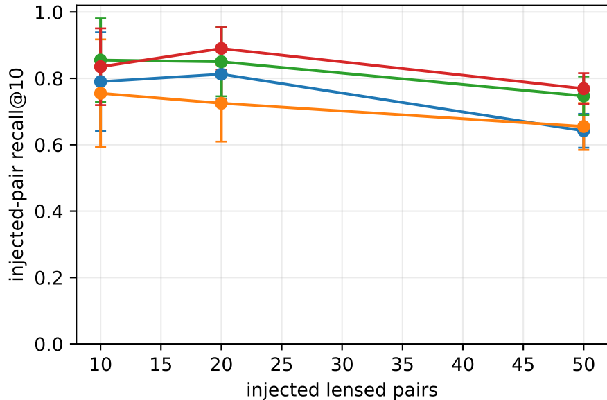
GWTC3
