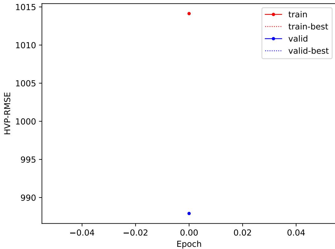
HVP-RMSE
