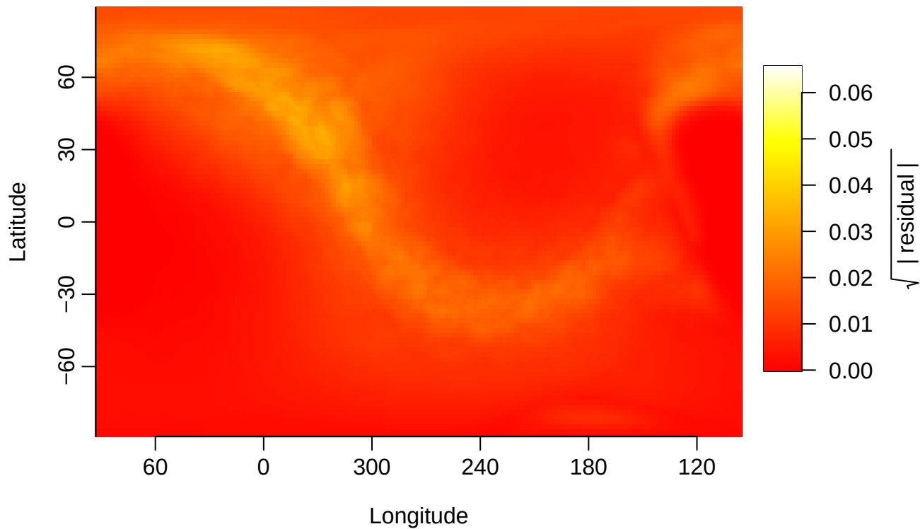
SEPIA ( n_k=3 )
