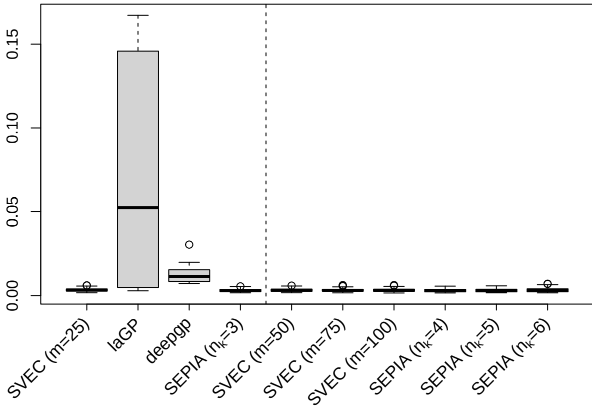
L-infinity distance
