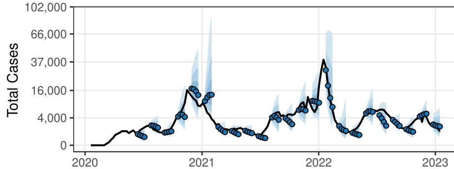
M(sv,v)
