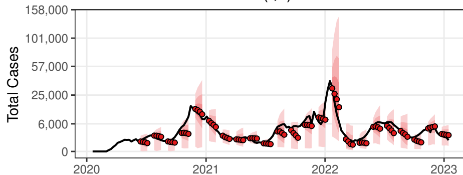
M(st,v)
