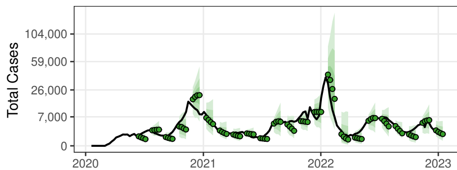
M(a,v)
