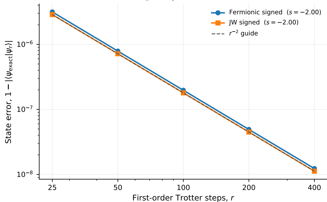
O 2 : 18 qubits (8+10)
