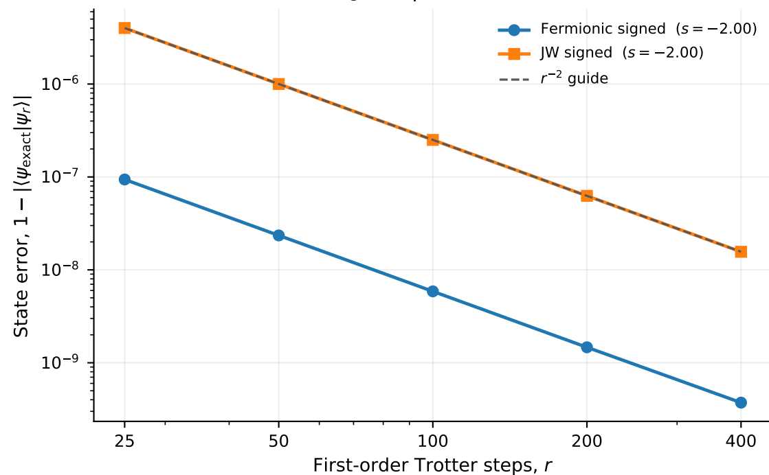
NH 3 : 18 qubits (8+10)
