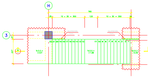
PLANTA ESCALERA 1°PISO a 2°PISO ESCALA 1:50
