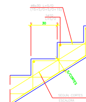
DETALLE ALTERNATIVO GRADAS ARMADAS ESCALA 1:10
