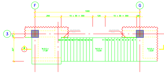
PLANTA ESCALERA 2°PISO a 3°PISO ESCALA 1:50
