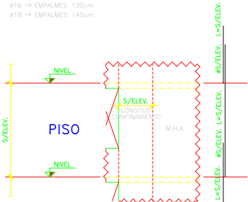
ELEVACIÓN MURO
