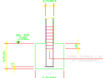
CORTE C
