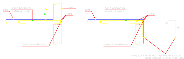
DETALLE ALTERNATIVO SUPLES EN MUROS ESCALA 1/25
