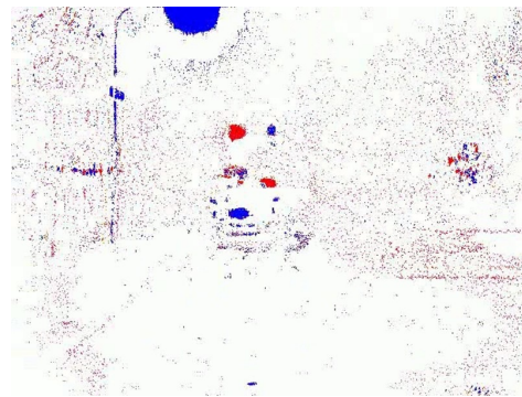
Ours
