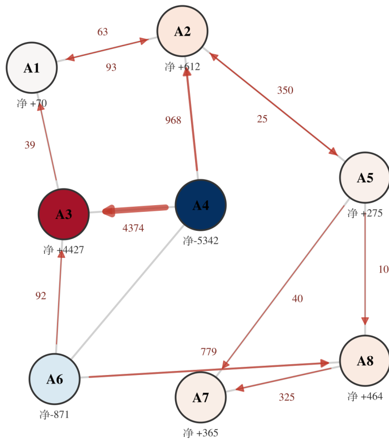
图 4 2025 年区域间电力碳流与净责任格局。箭头宽度正比于到达碳量 F_{j \rightarrow i} ( \text{ktCO}_2 )；节点颜色为 C_i^+ - P_i^+ (红 = 净转入)。主路径为 A4 → A3 (4374 kt)。
