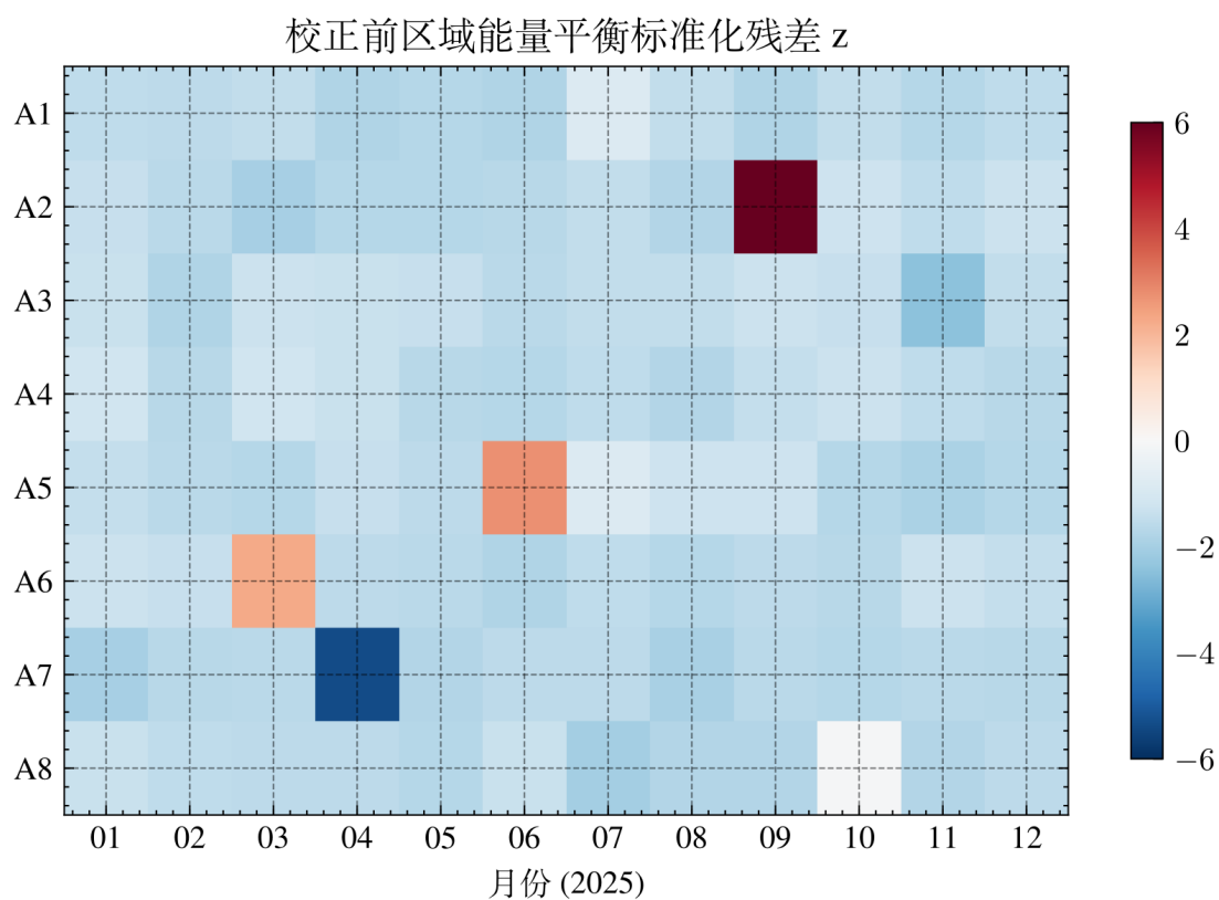
图1 校正前各区域—月份能量平衡标准化残差。颜色为 z_{i,t} = r_{i,t}/\sigma_{i,t} ; |z| > 3 对应 A2 九月等粗差。
