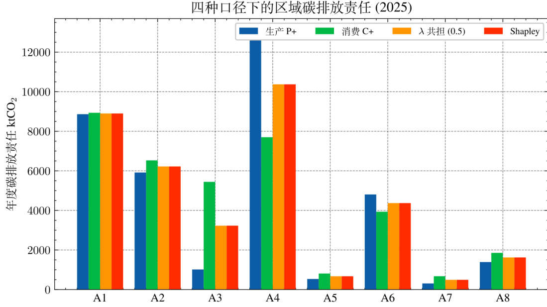
图 5 四种口径下的区域碳排放责任 (2025)。λ = 0.5 与 Shapley 柱高重合，验证五五分成的博弈含义。
