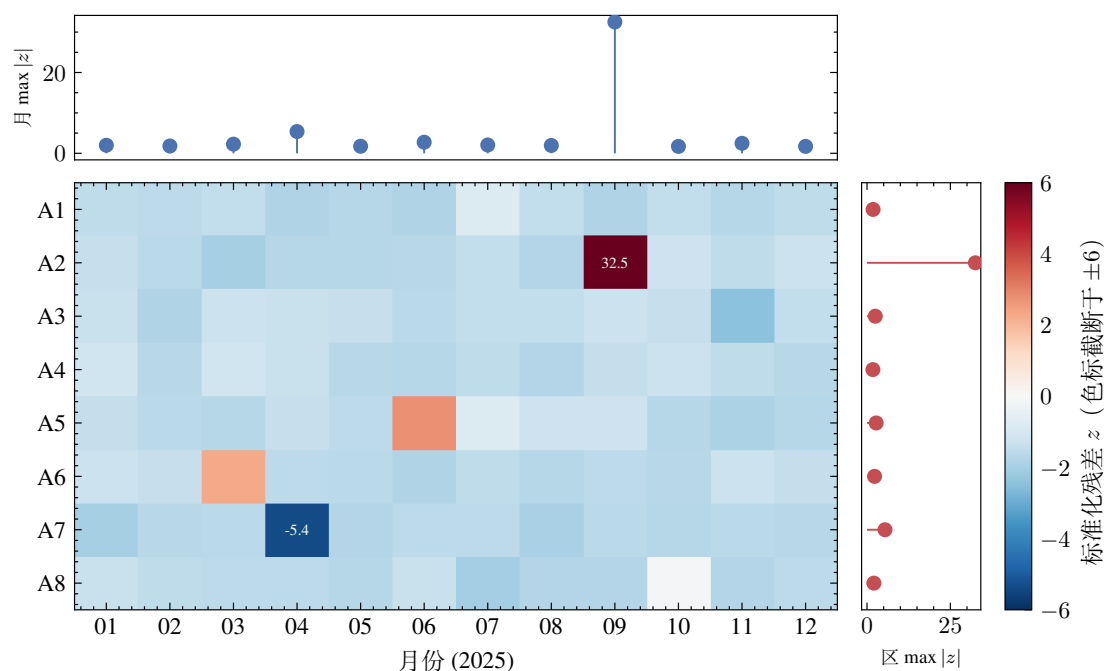
图 2 校正前能量平衡标准化残差。色标截断于 \pm 6 ，边际条为各月、各区的 \max |z| ；A2 九月初端值 z = 32.5 另行标明。
