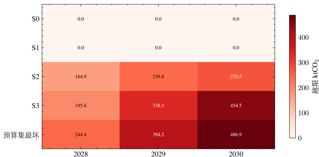
图 15 问题三加权罚基线的越限热力图(情景 \times 年份)。S0 均为零, S3 情景下 2030 年为 454.5 kt。
