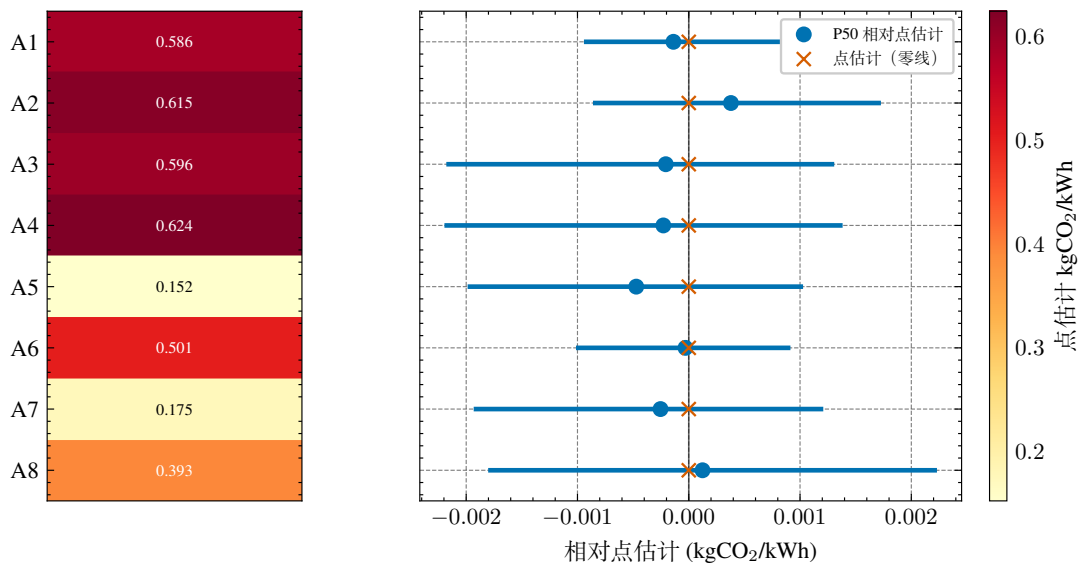
图 11 八区域年均终端碳强度点估计及 95% 条件区间。右图采用相对偏差轴，圆点为 P50。
