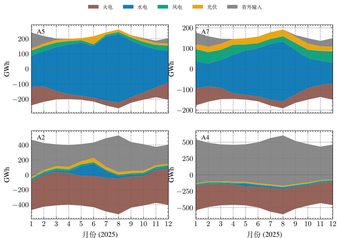
图7 典型区域逐月电源结构对称流图。带宽正比于终端电量、中线为零；A5/A7 丰水期水电变宽，A2 火电、A4 省外输入全年占优。
