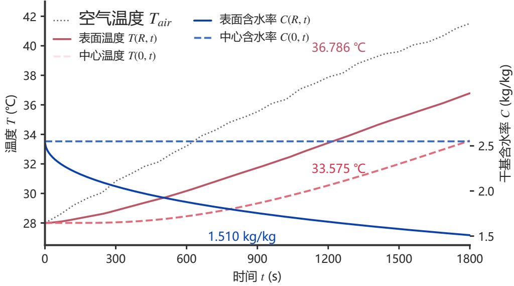
图 7 问题一中心与表面测点的时程对照
