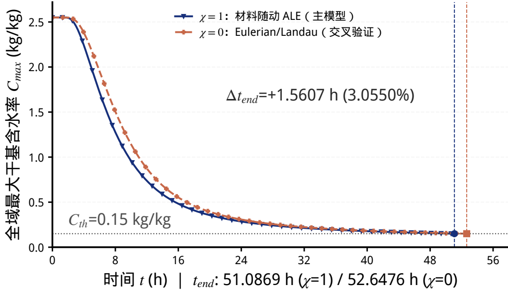
图 18 问题四移动边界闭合方式的最终时程对比
