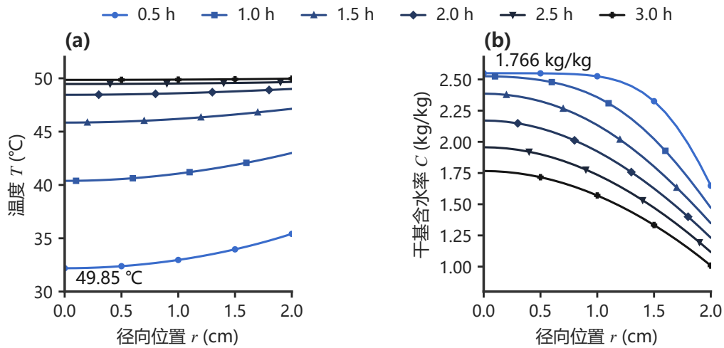
图 9 问题二温度与含水率的径向剖面
