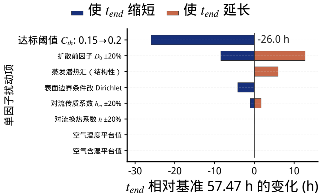
图 20 达标时长的最终精度单因子灵敏度诊断
