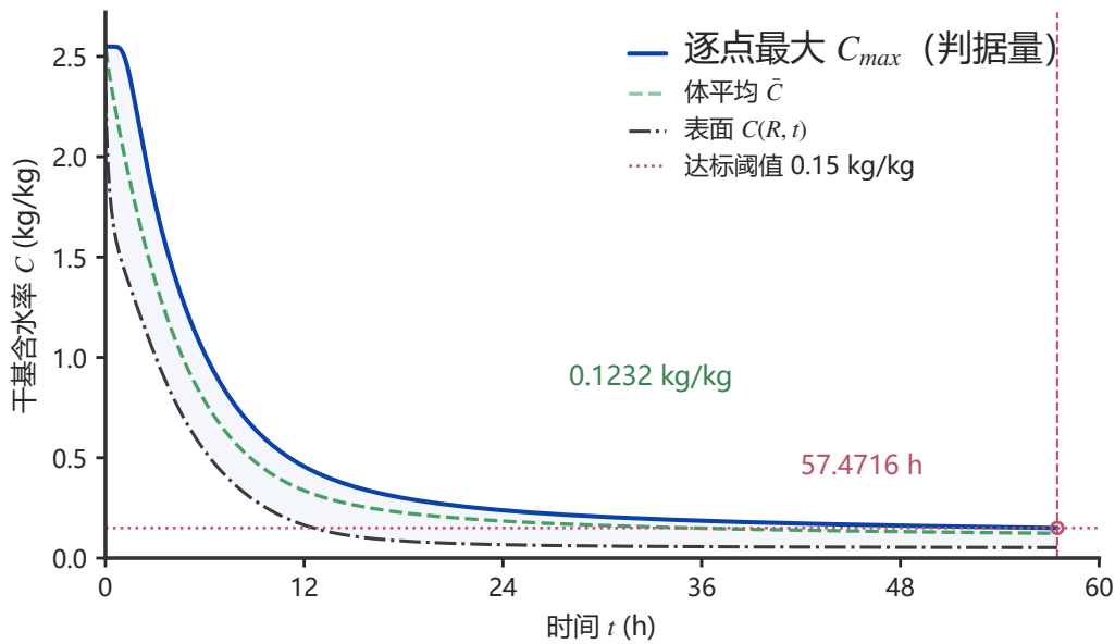
图 11 问题三干燥曲线与达标时刻定位
