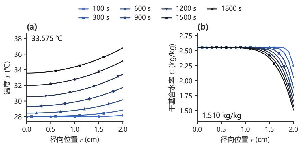
图 6 问题一温度与含水率的径向剖面
