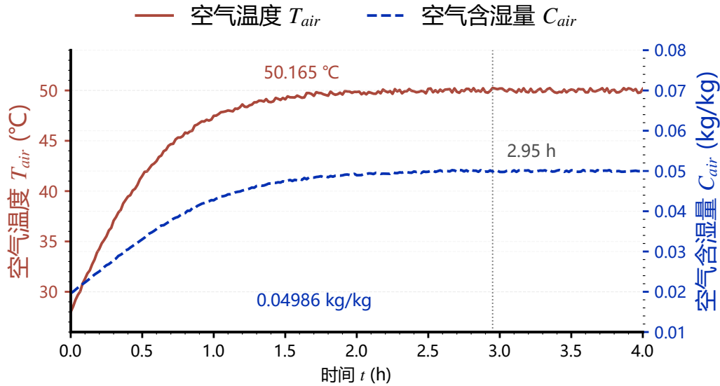
图 3 附件 1 干燥室工况的双轴时程
