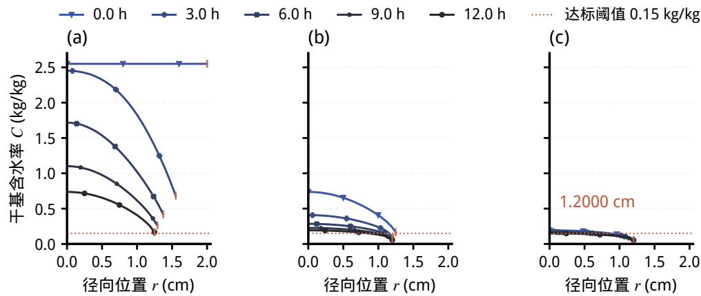
图 16 问题四含水率剖面的三阶段演化
