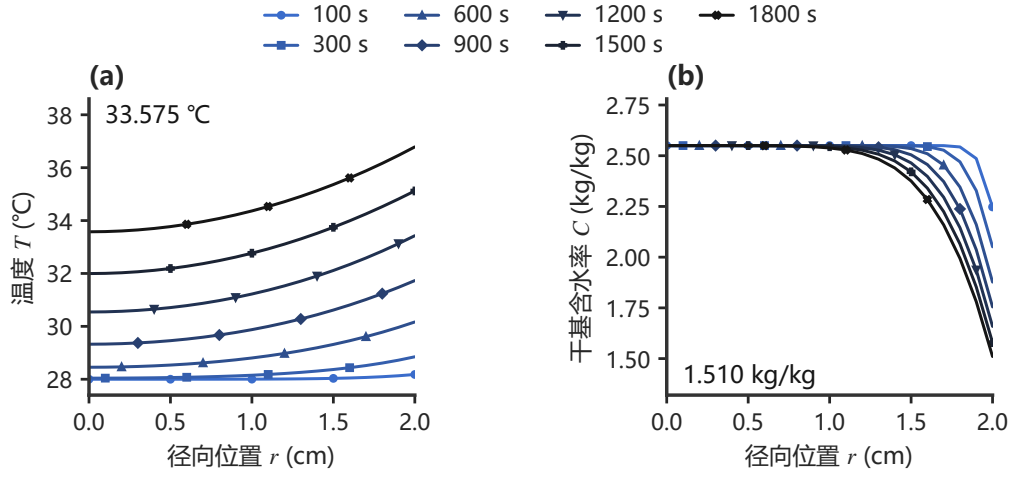
图 6 问题一温度与含水率的径向剖面
