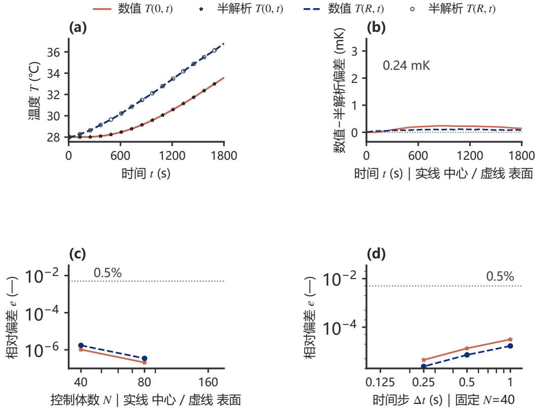
图 8 问题一数值解的四项校核证据
