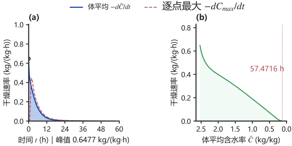
图 12 问题三干燥速率的两种读法
