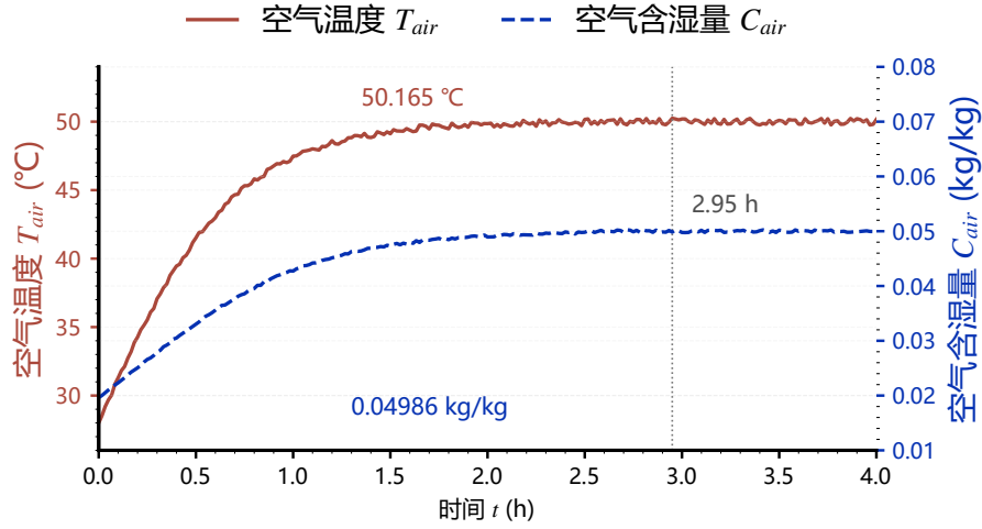
图3 附件1干燥室工况的双轴时程
