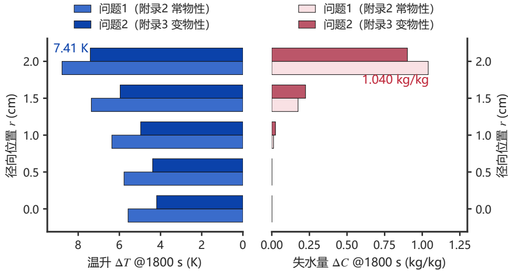
图10 问题一与问题二在 t = 1800 \text{ s} 的增量对比
