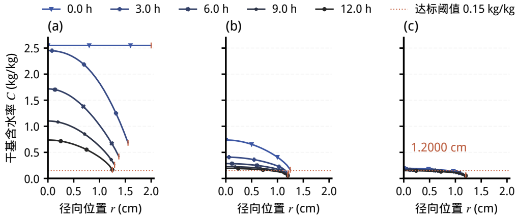
图 16 问题四含水率剖面的三阶段演化
