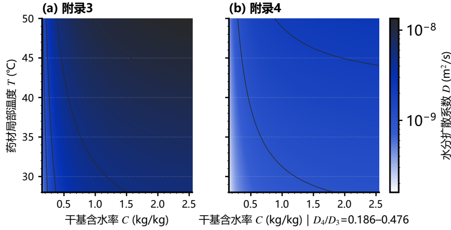
图 4 附录 3 与附录 4 的水分扩散系数分布对比
