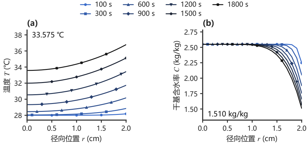
图 6 问题一温度与含水率的径向剖面
