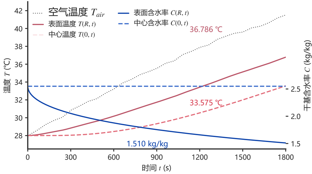
图 7 问题一中心与表面测点的时程对照
