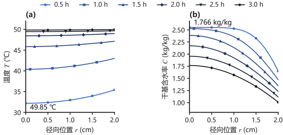
图9 问题二温度与含水率的径向剖面
