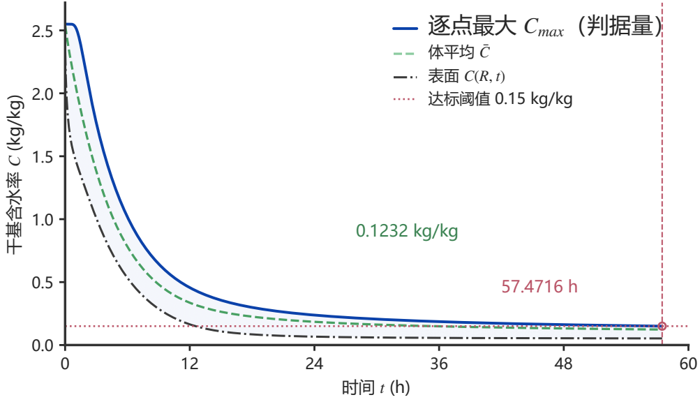
图 11 问题三干燥曲线与达标时刻定位
