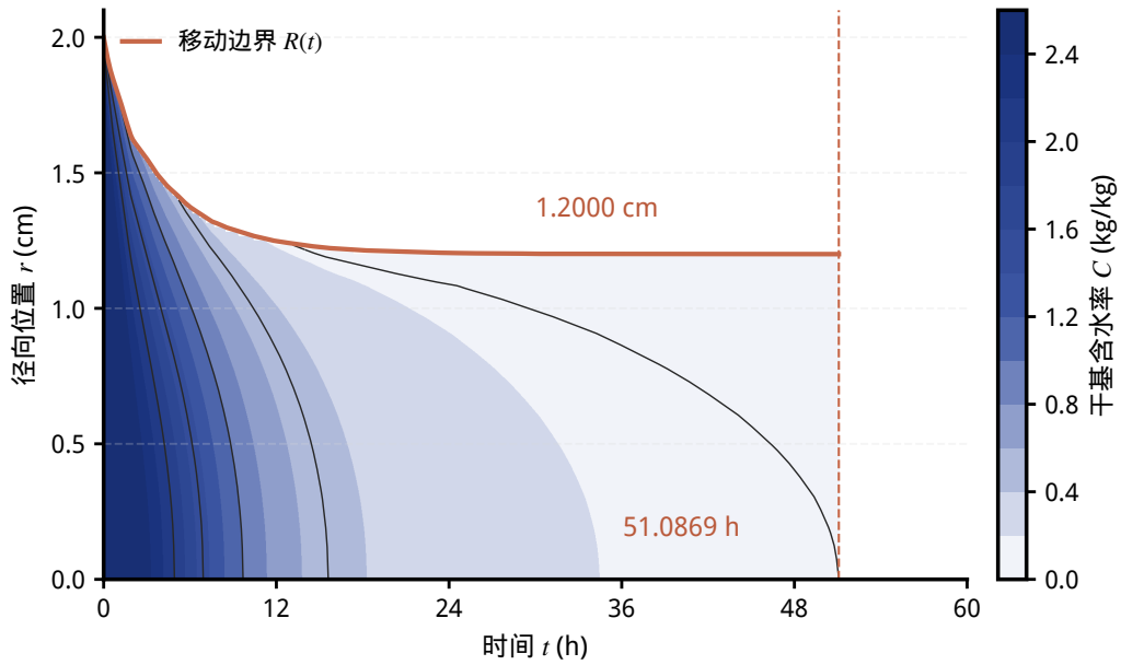
图 19 问题四收缩域内含水率的时空分布与移动边界
