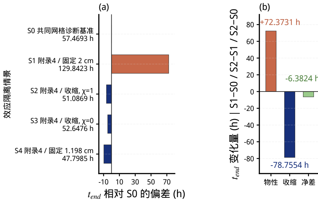
图 22 问题四的效应隔离与加性分解（共同网格诊断）
