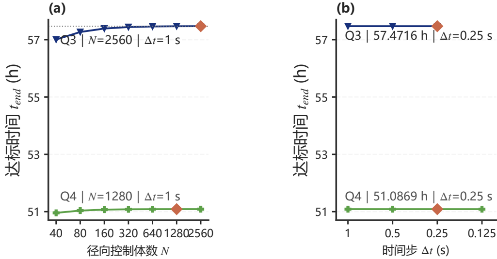
图 25 问题三与问题四的空间和时间步收敛性
