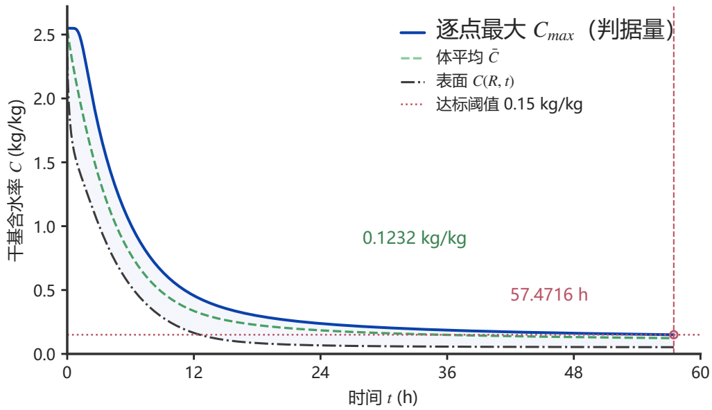
图 15 问题三干燥曲线与达标时刻定位
