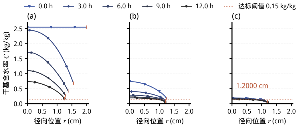
图 20 问题四含水率剖面的三阶段演化
