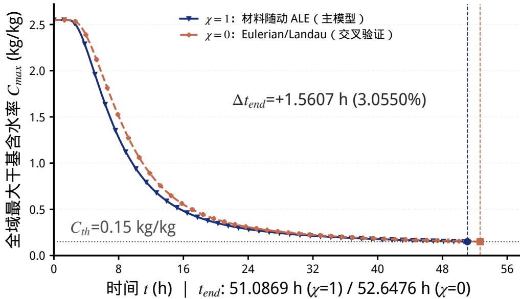
图 23 问题四移动边界闭合方式的最终时程对比
