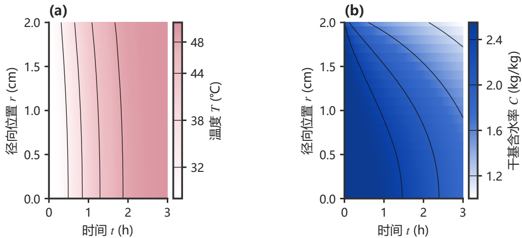
图 12 问题二温度场与含水率场的时空分布
