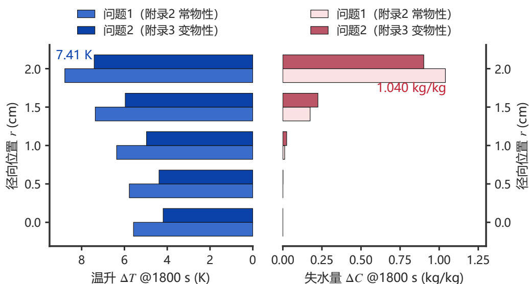
图 13 问题一与问题二在 t = 1800 \text{ s} 的增量对比
