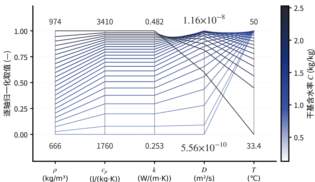
图 14 附录 3 四项物性随含水率的联动
