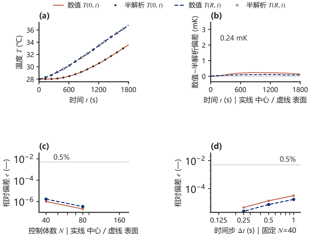
图 10 问题一数值解的四项校核证据
