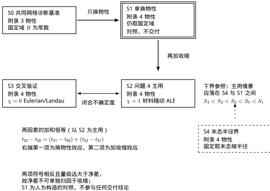
图 21 问题四相对问题三的两因素效应隔离路径
