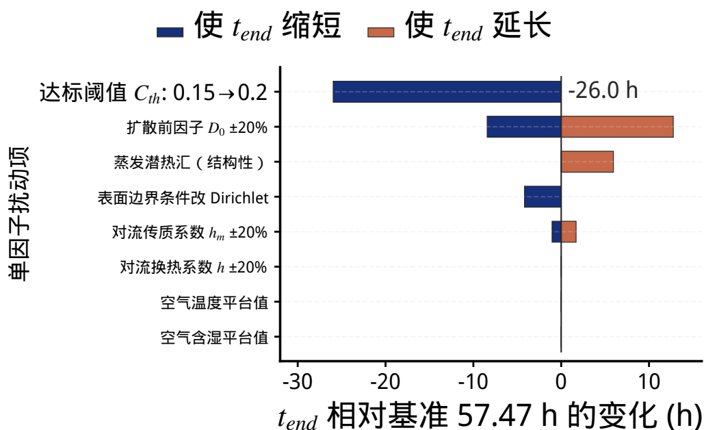
图 26 达标时长的最终精度单因子灵敏度诊断
