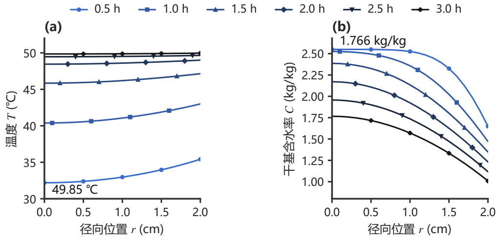
图 11 问题二温度与含水率的径向剖面
