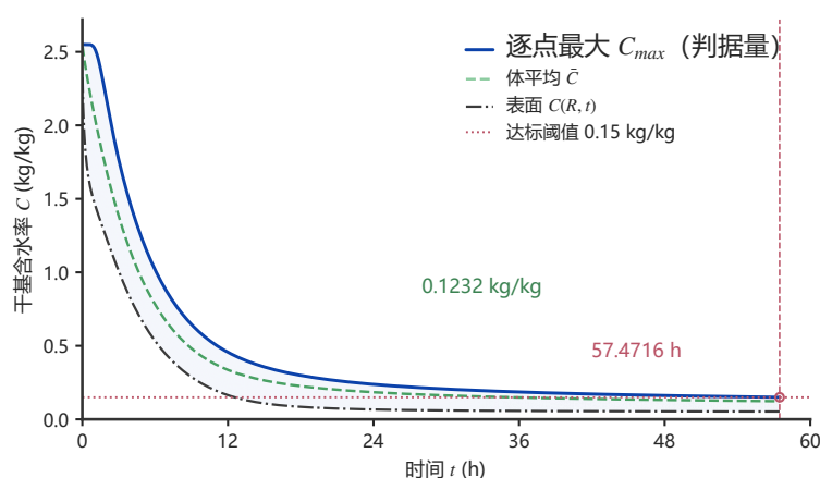
图 11 问题三干燥曲线与达标时刻定位
