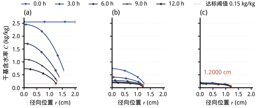
图 16 问题四含水率剖面的三阶段演化
