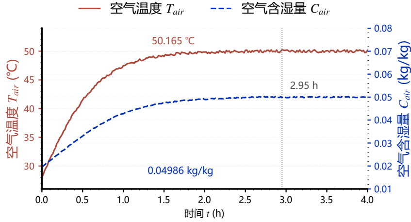
图3 附件1干燥室工况的双轴时程
