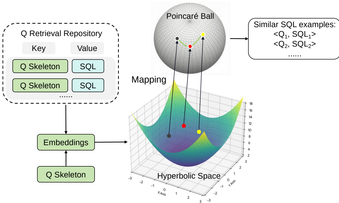
图 5.4 庞加莱球示例选择
