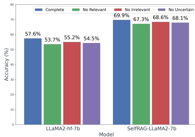
图 4.6 移除了 Arc-Challenge 数据集上每个单独动作的消融研究（准确率%）
