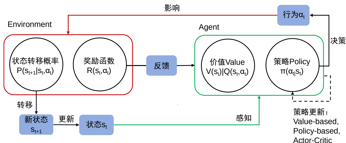
图 2.1 强化学习的一般性框架示意图
