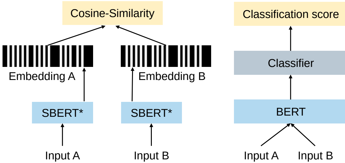
图 2.2 Bi-Encoder（左）和 Cross-Encoder（右）
