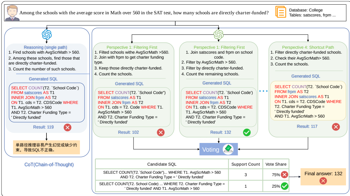
图 3.1 NL2SQL 任务中用户意图识别错误示例
