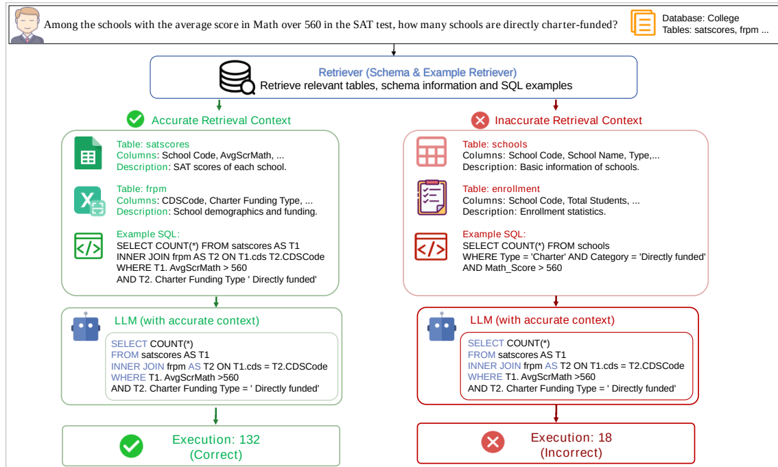
图 4.1 NL2SQL 知识检索中的低质量检索器引入噪声信息示例
