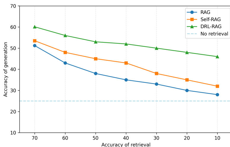
图 4.7 基模型 SelfRAG-Llama-7b 在 PopQA 上的检索准确率下降与生成性能差异分析
