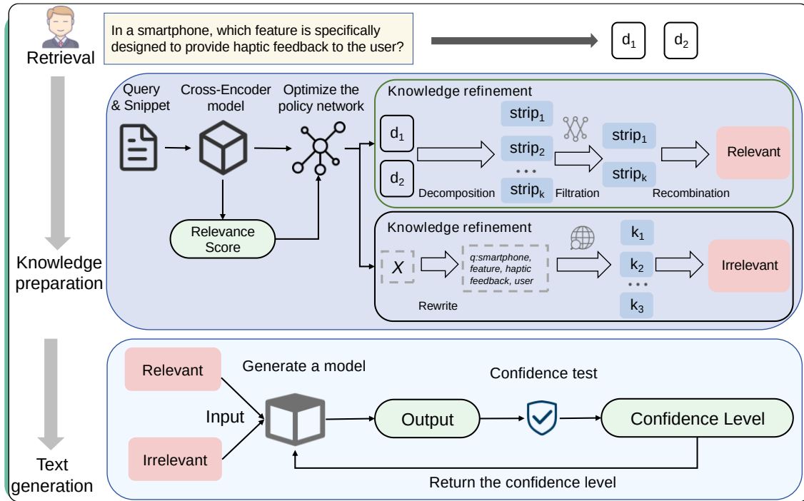
图 4.2 基于强化学习的自适应检索与置信度感知生成
