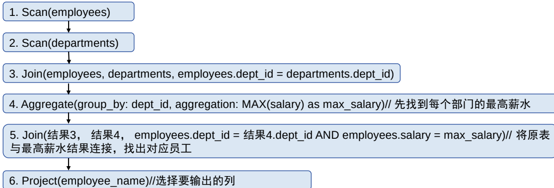
图 3.3 逻辑计划生成
