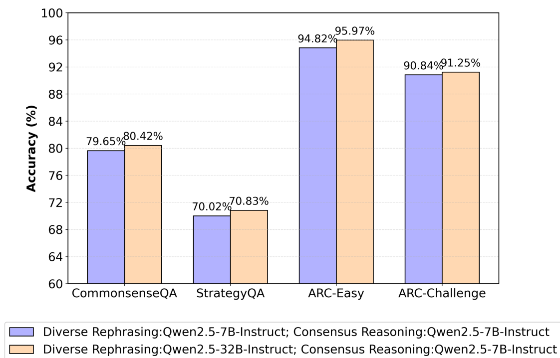
图 3.4 不同参数规模的大语言模型在协同推理中的效应
