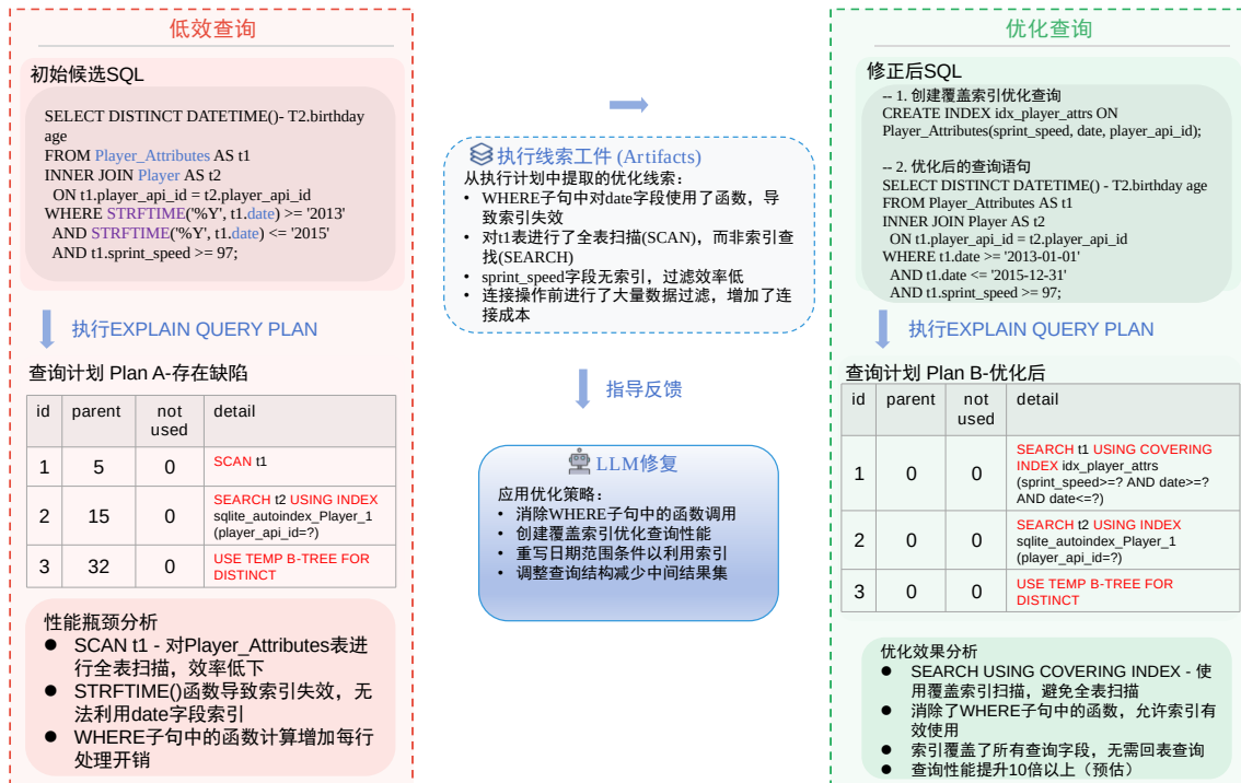
图 5.5 从 BIRD [9] 数据集的 european_football_2 数据库中选择的查询计划优化 SQL 示例
