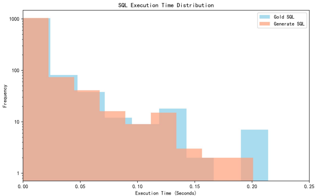
图 5.7 生成 SQL 和 Gold SQL 的执行时间分布
