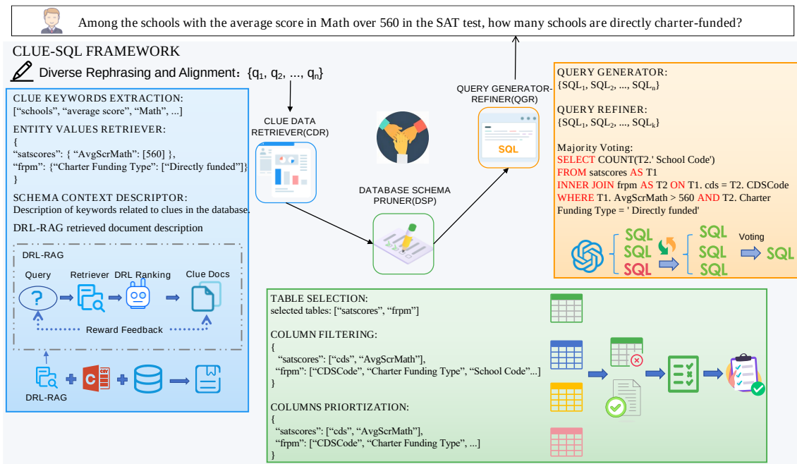
图 5.1 用于 NL2SQL 任务的 CLUE-SQL 多智能体框架包括三个代理：线索数据检索代理 (CDR)、数据库模式剪枝代理 (DSP) 和生成器优化代理 (QGR)
