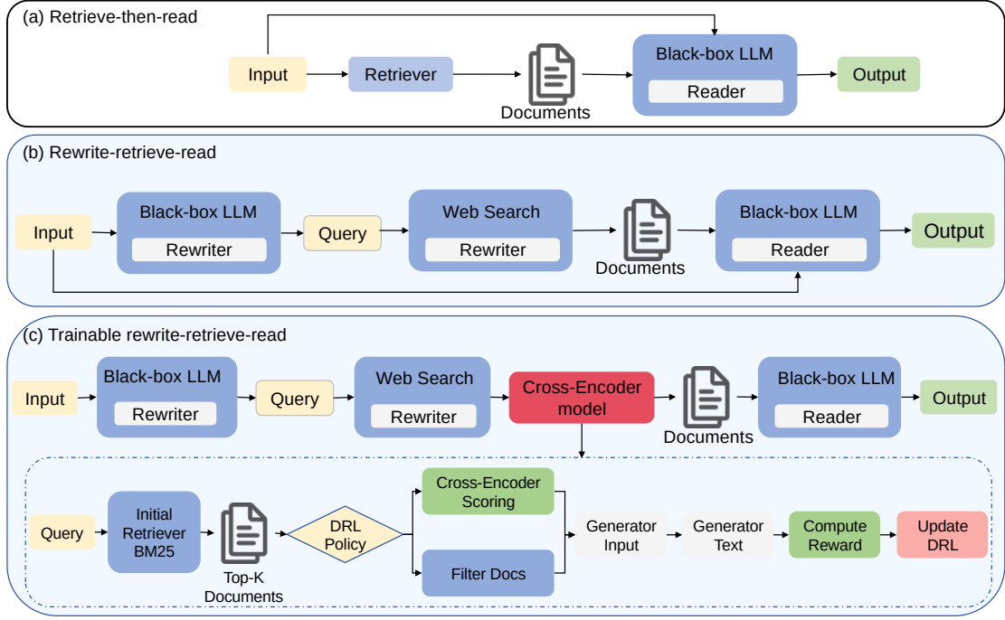
图 4.3 概述我们提出的管道，比较三个阶段：(a) 标准检索然后读取，(b) 基于 LLM 的查询重写，以及 (c) 集成可训练的重写器
