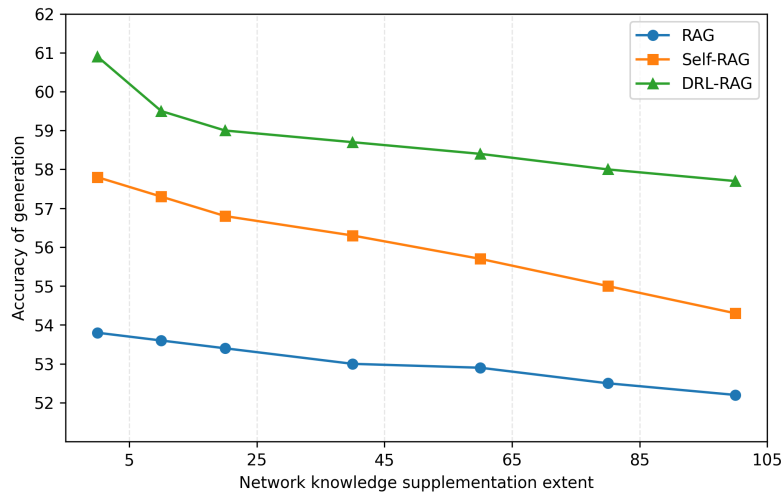
图 4.8 基模型 SelfRAG-Llama-7b 在 PopQA 上的网络知识补充效果减弱与生成性能分化
