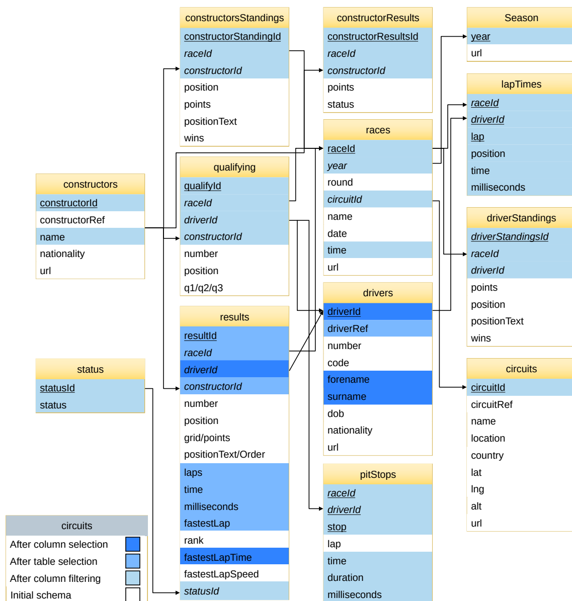
图 5.3 模式选择示例 formula_1_926
