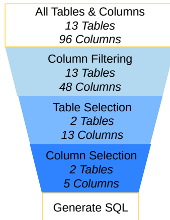
图 5.2 基于代理剪枝的数据库模式逐步筛选流程
