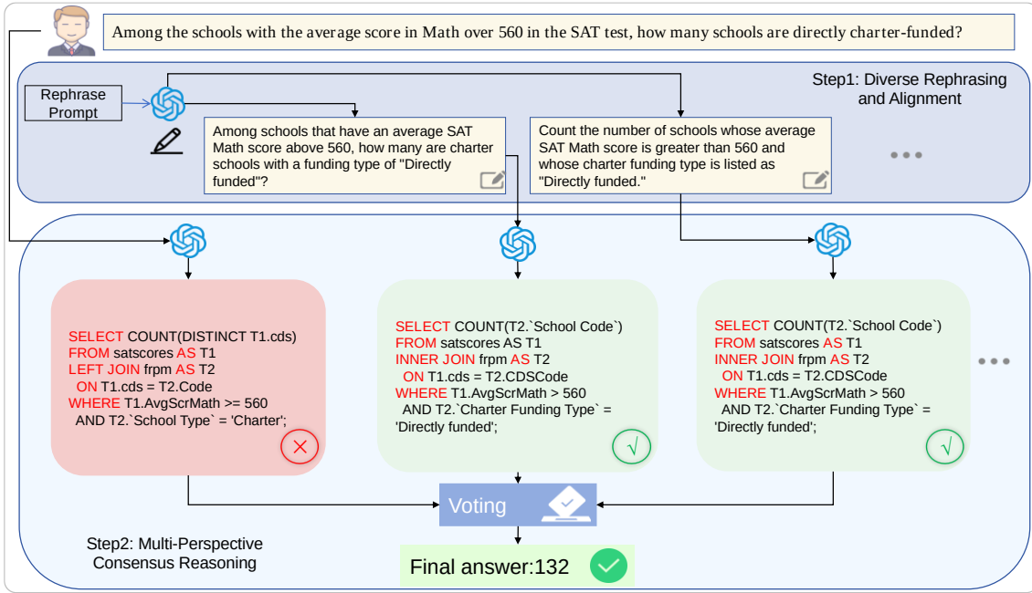
图 3.2 认知对齐推理 (CAR) 方法
