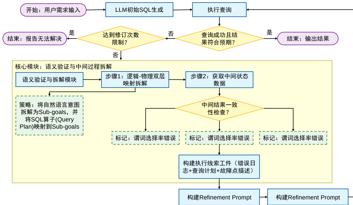
图 5.6 利用中间状态对齐与子目标拆解的 SQL 故障定位及修复机制
