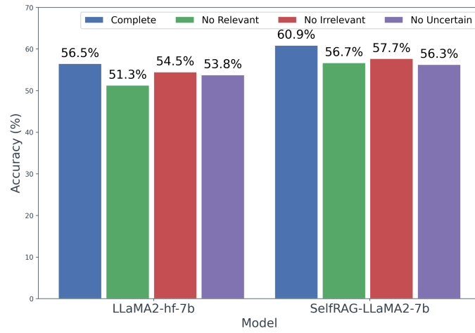
图 4.4 移除了 PopQA 数据集上每个单独动作的消融研究（准确率%）
