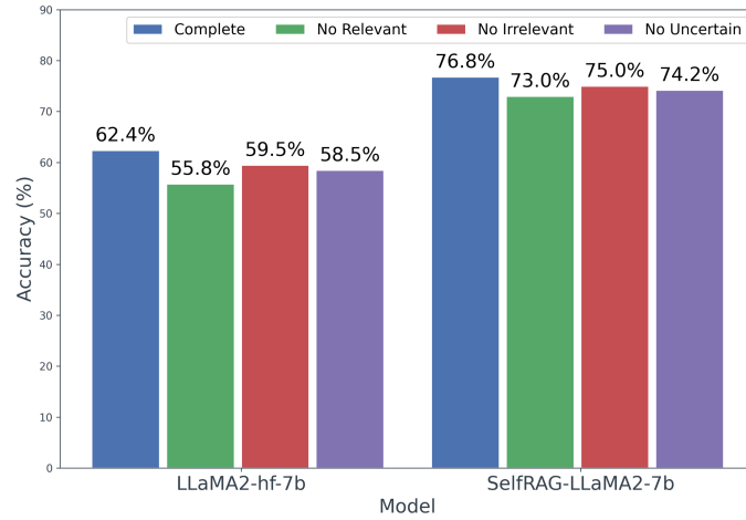
图 4.5 移除了 PubHealth 数据集上每个单独动作的消融研究（准确率%）
