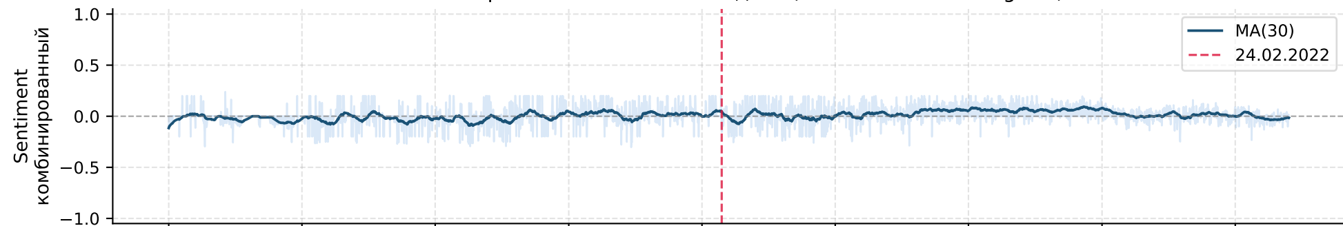
Комбинированный sentiment-индекс (RSS + GDELT + Telegram)
