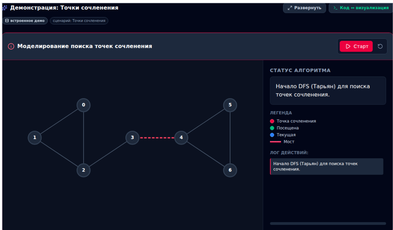
Точки сочленения
