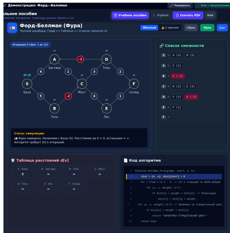
Форд—Беллман
