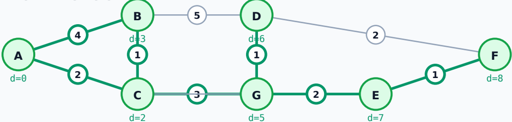
Векторный граф релаксации (Дейкстра)
