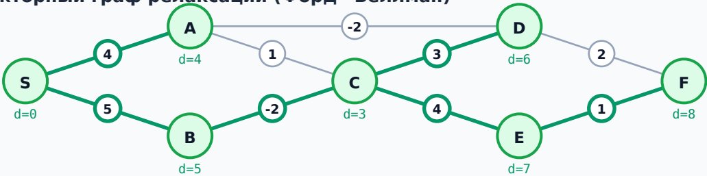
Векторный граф релаксации (Форд—Беллман)
