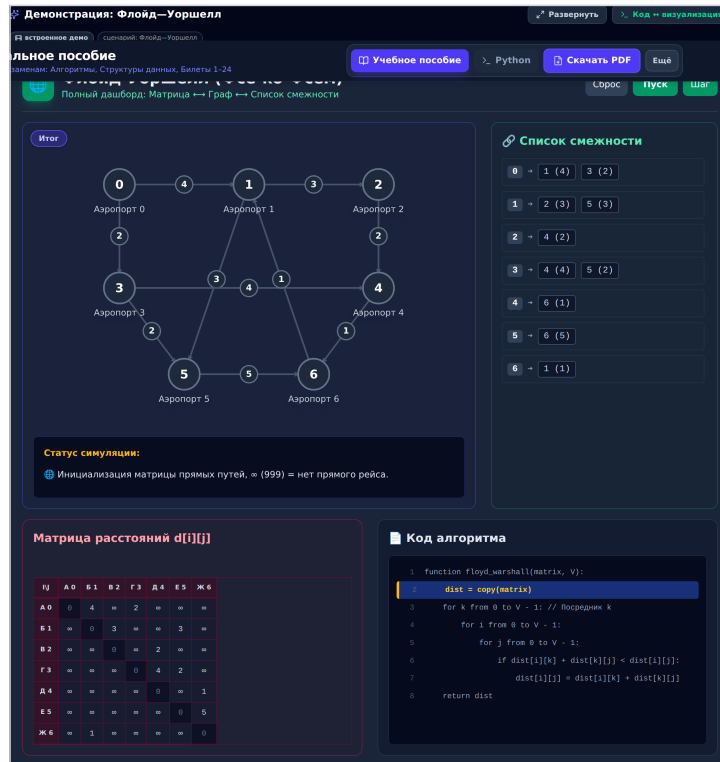
Флойд—Уоршелл
