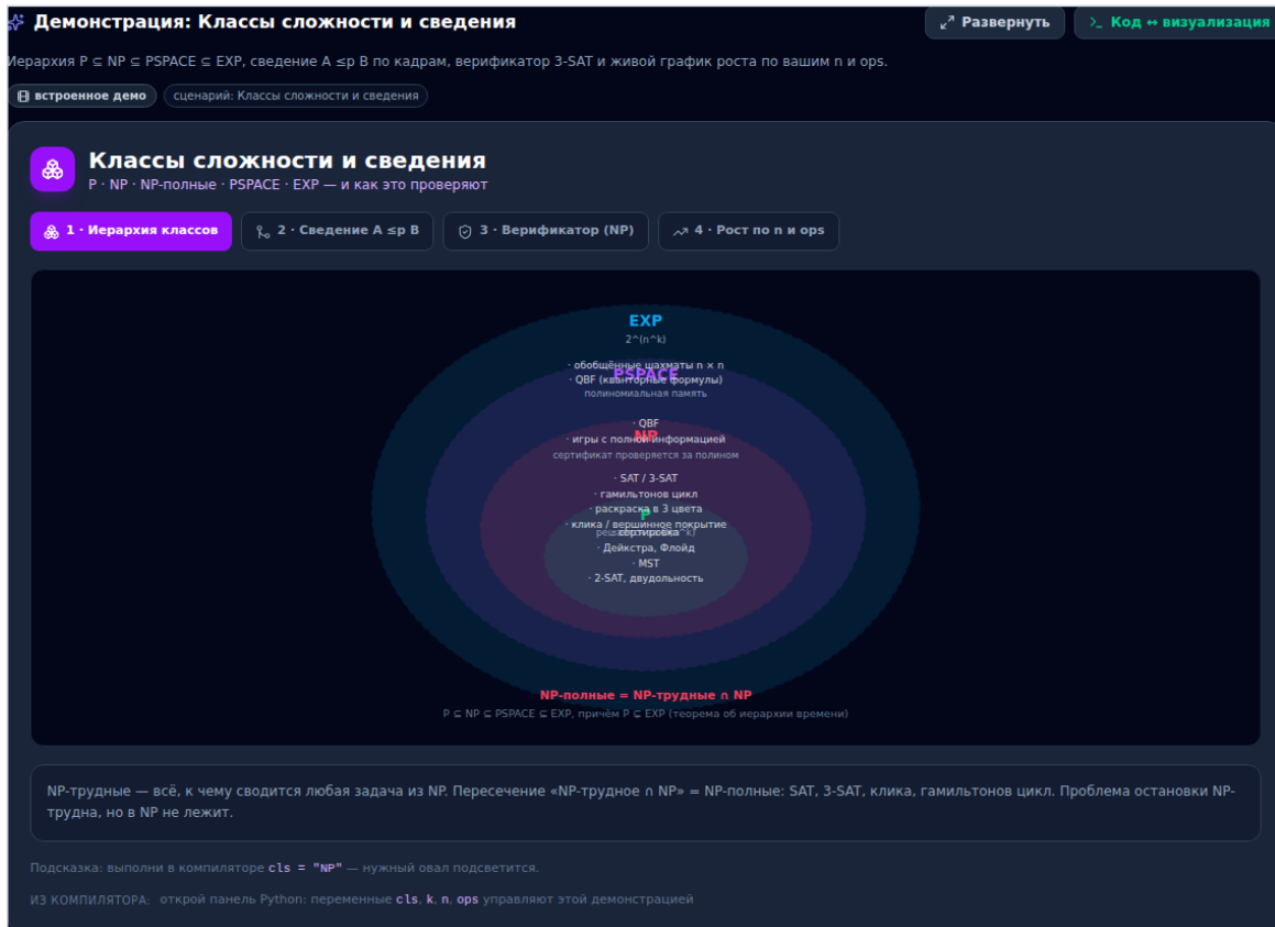
Классы сложности и сведения
