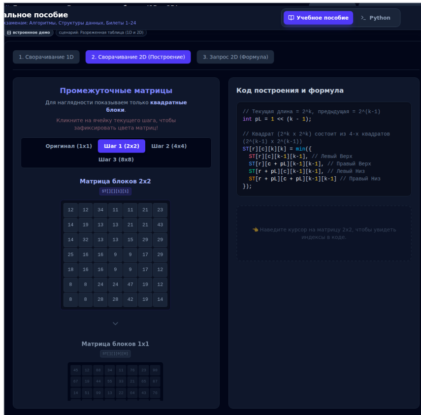
Разреженная таблица (1D и 2D)
