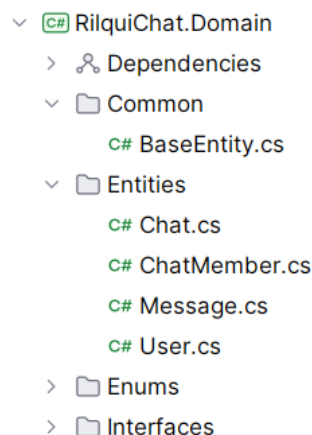
Рисунок 3.2 – Структура доменного слоя
