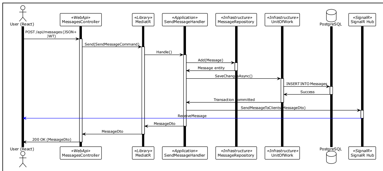
Рисунок 3.6 – Диаграмма последовательности для отправки сообщения
