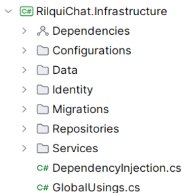
Рисунок 3.4 – Структура слоя инфраструктуры
