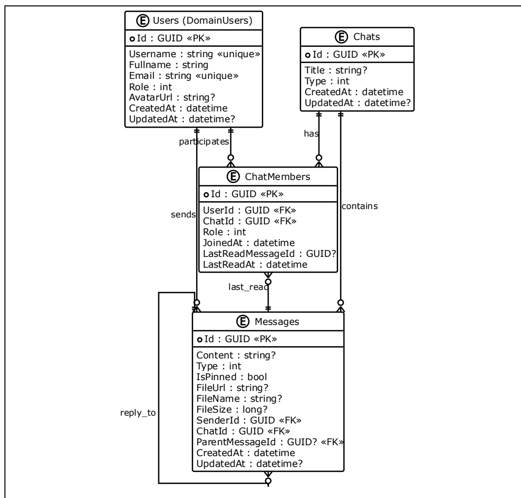
Рисунок 3.8 – ER-диаграмма базы данных
