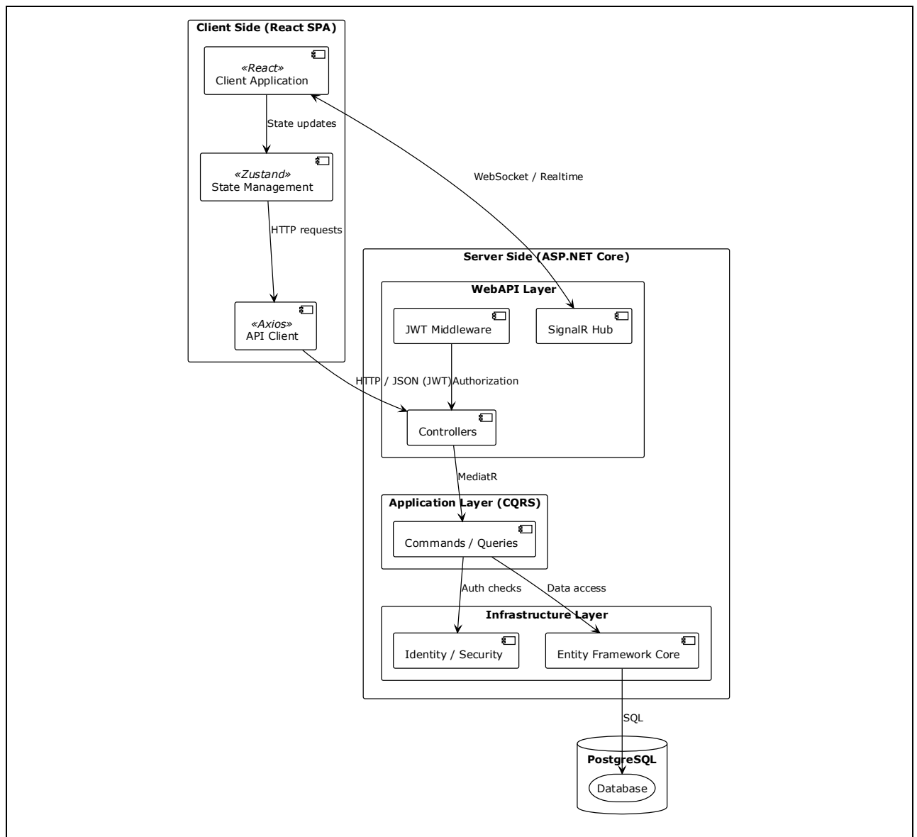
Рисунок 3.1 – Структура программного комплекса корпоративного мессенджера
