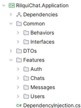
Рисунок 3.3 – Структура слоя приложения
