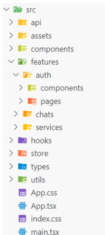
Рисунок 3.9 – Структура клиентской части
