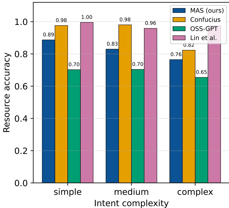
gpt-oss:120b
