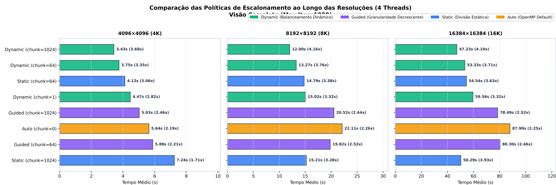
Figura 7 – Comparação das políticas de escalonamento ao longo das resoluções na Visão Completa.
