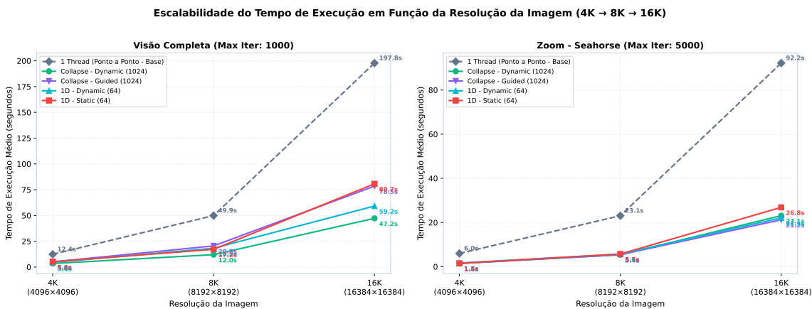
Figura 10 – Escalabilidade do tempo de execução em função da resolução da imagem (4K → 8K → 16K).
