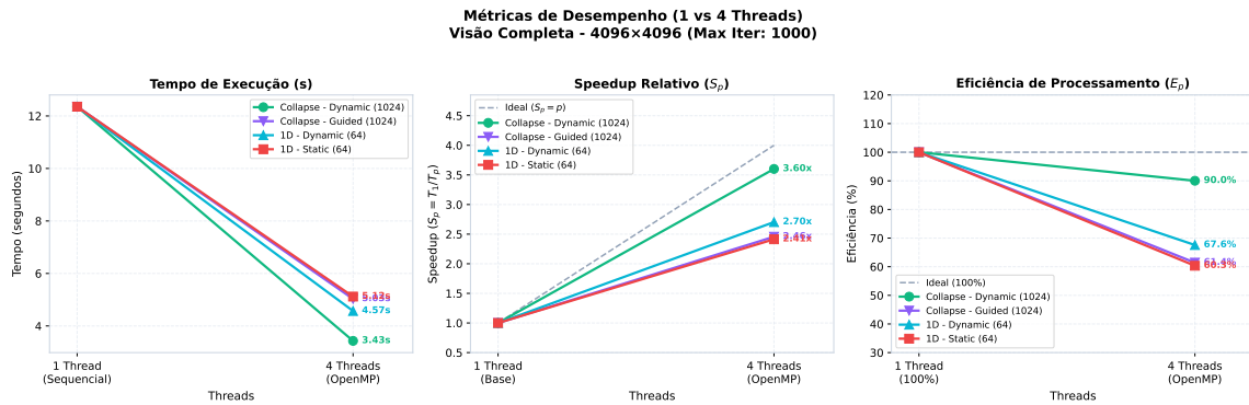
Figura 3 – Escalabilidade e métricas de aceleração entre 1 e 4 threads no cenário padrão.
