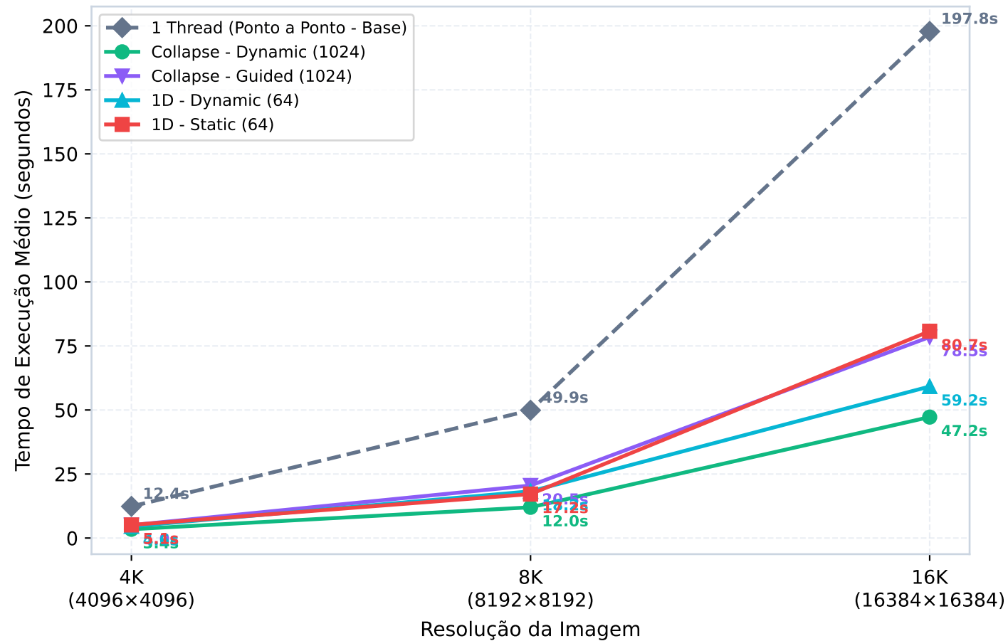
Visão Completa (Max Iter: 1000)
