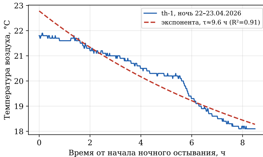
Рисунок 3.12 – Ночное остывание датчика th-1 и экспоненциальный фит первого порядка (идентификация постоянной времени теплового баланса)
