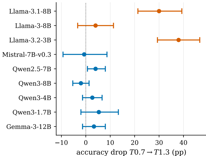
GSM8K
