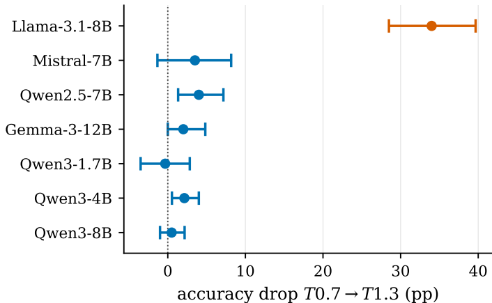
GSM8K
