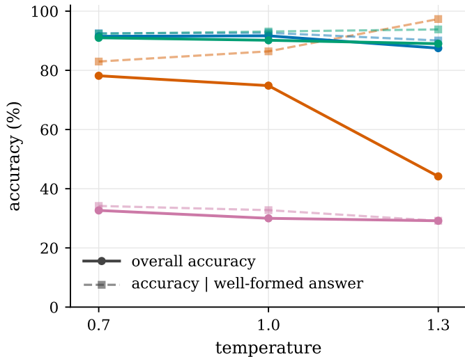
GSM8K
