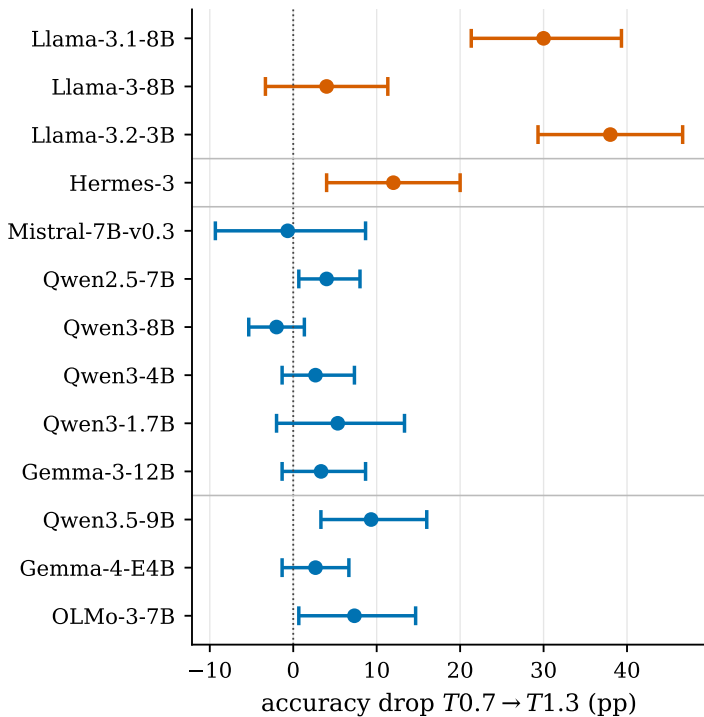
GSM8K
