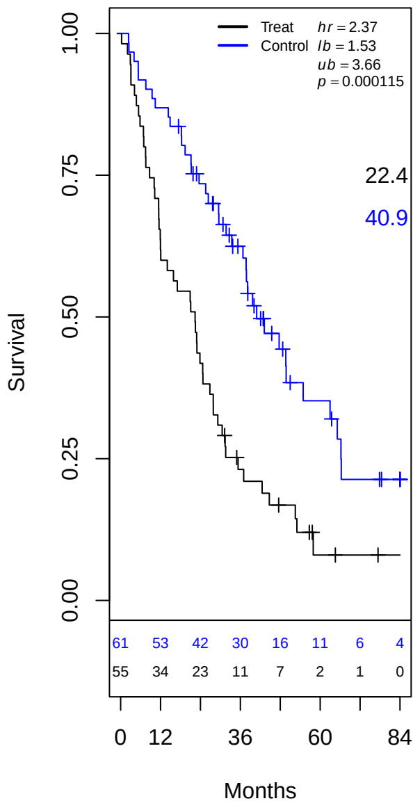
!{z3 <= 0} & {z1}
