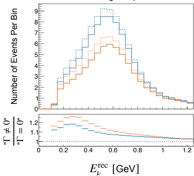
FHC 1e -Ring Sample – MC
