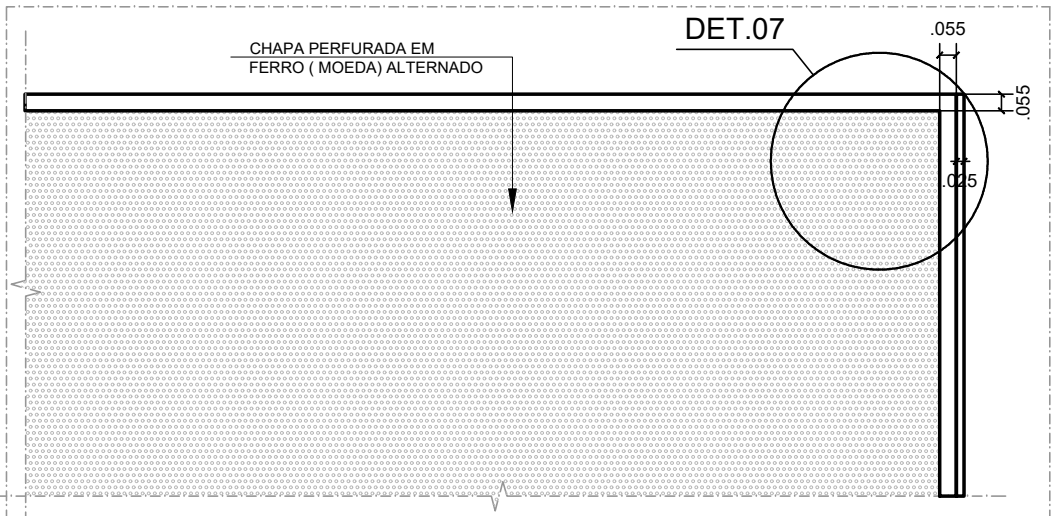
DET.07- VISTA DA CHAPA PERFORADA ESCALA 1:25
