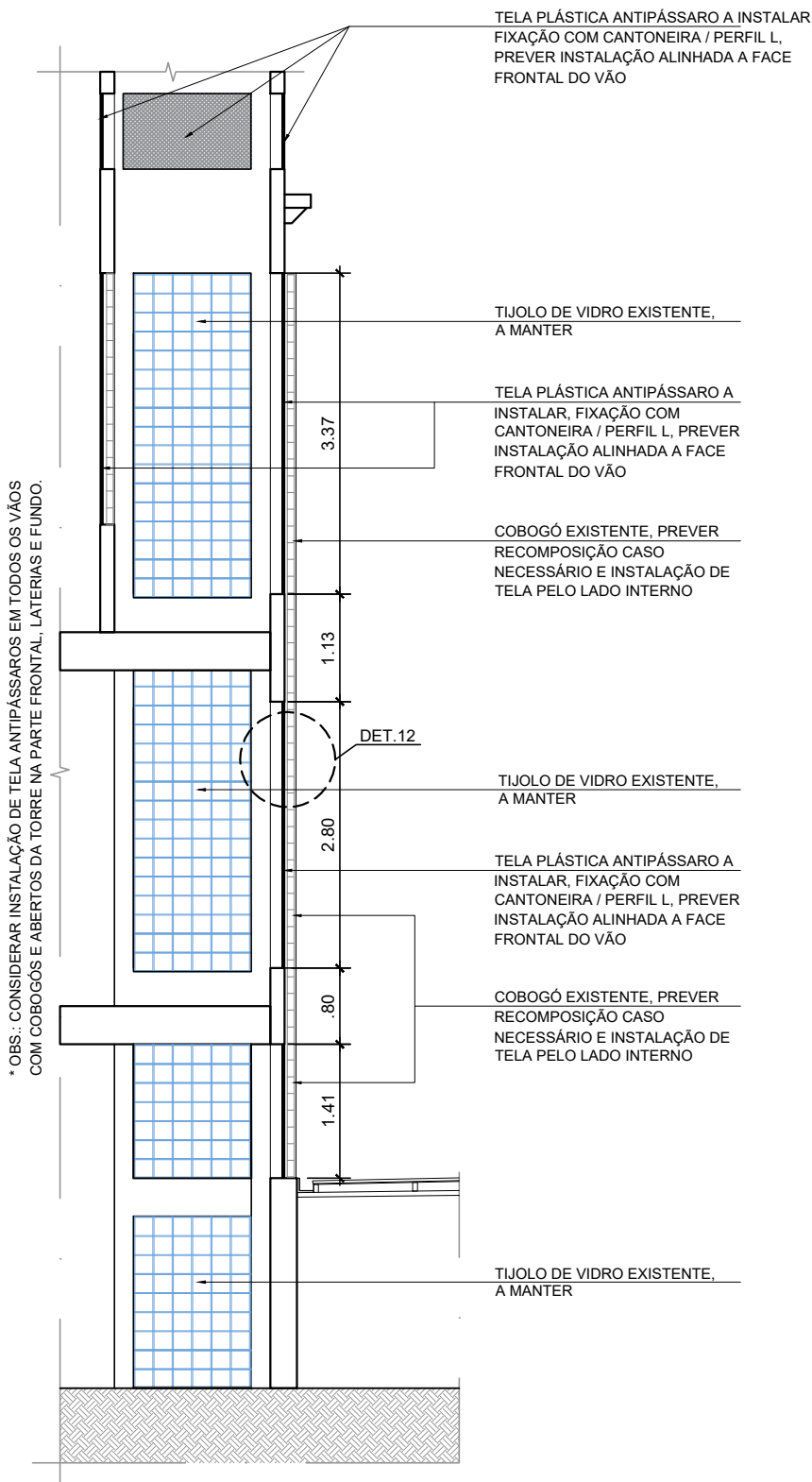
CORTE E-E ESCALA 1:75
