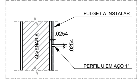
DET. 02 ESCALA 1:25
