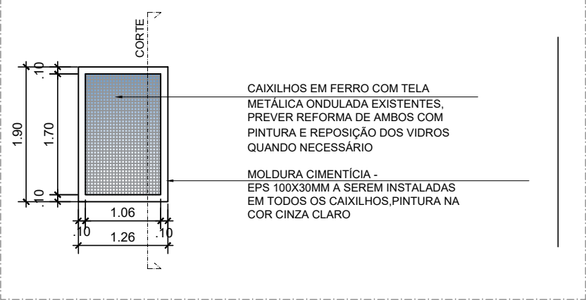
DET. 09 VISTA 3 ( COM TELA METÁLICA ) ESCALA 1:75
