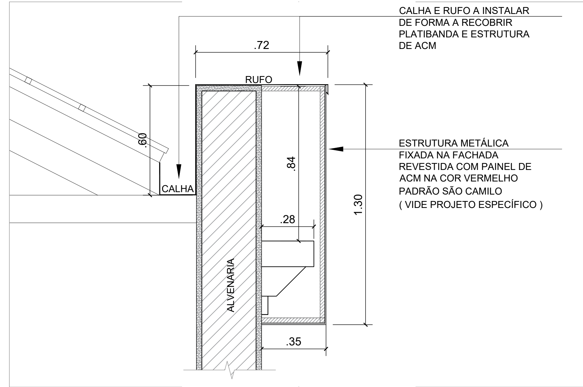
DET. 03- ORIENTATIVO ESCALA 1:25
