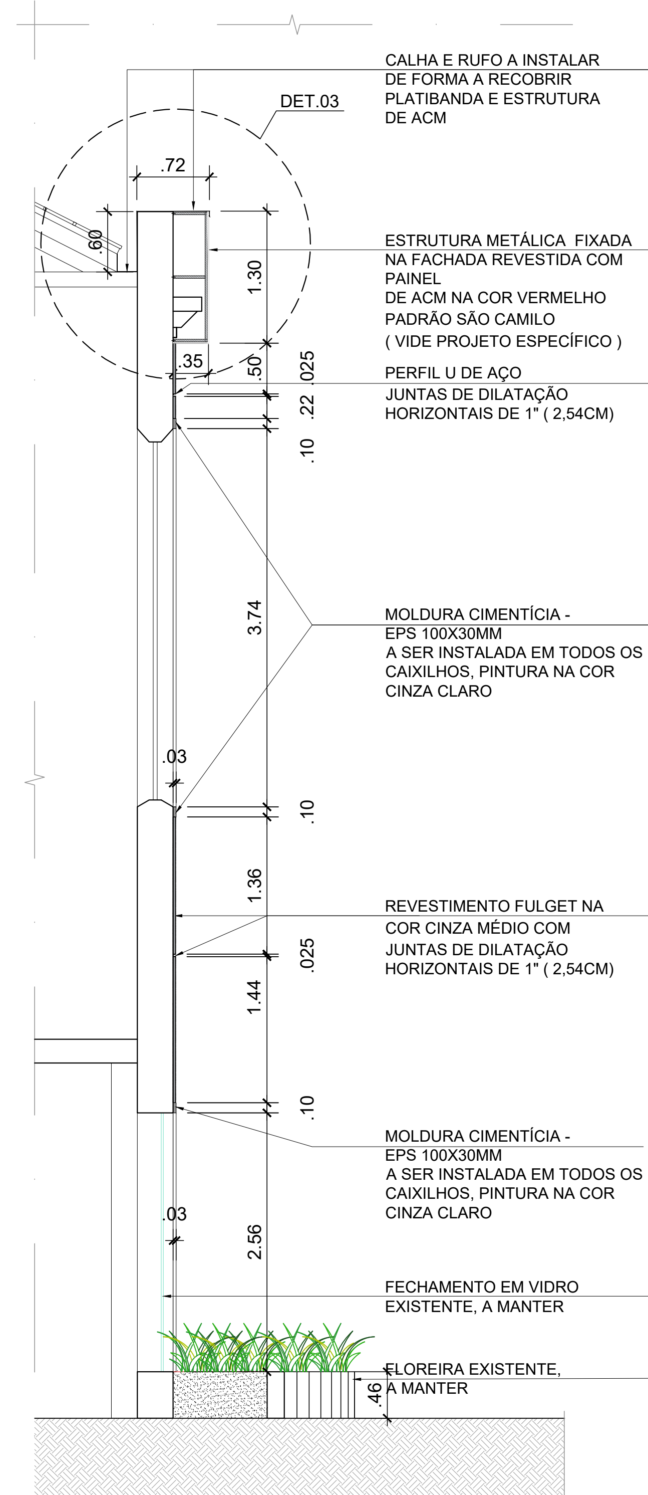
CORTE H-H ESCALA 1:75
