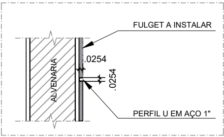
DET. 02 ESCALA 1:25
