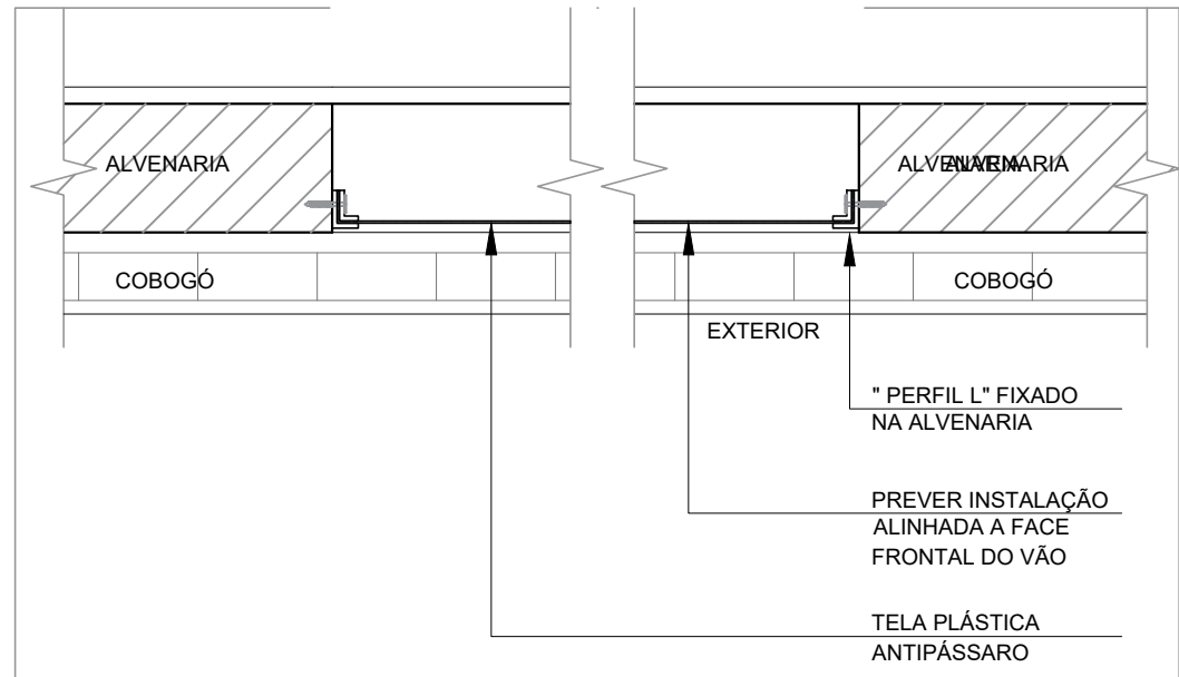
DET. 12 ESCALA 1:25
