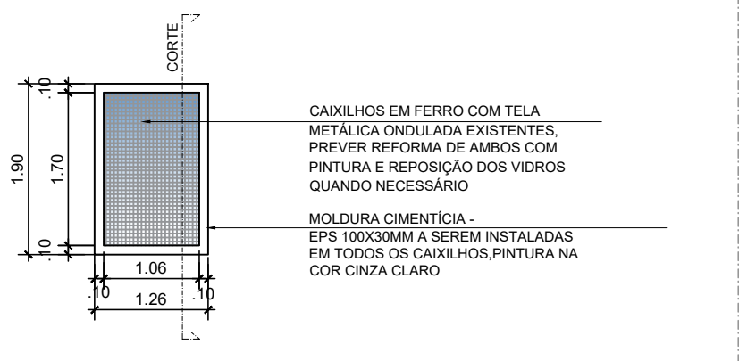
DET. 09- VISTA 5 ( COM TELA METÁLICA ) ESCALA 1:75
