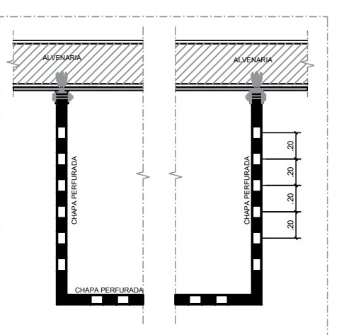
DET. 07 GENÉRICO FIXAÇÃO DA CHAPA PERFORADA ESCALA 1:25
