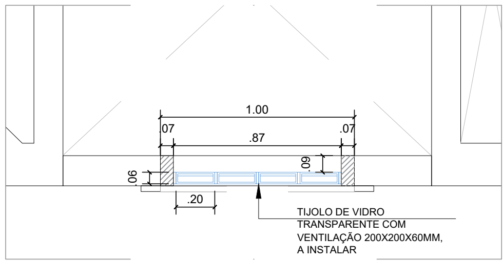
DET. 11- PLANTA ( TIJOLO DE VIDRO ) ESCALA 1:25
