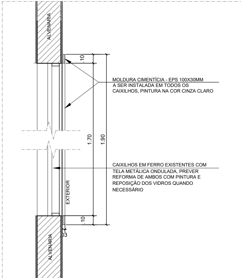
DET. 09 CORTE ( COM TELA METÁLICA ) ESCALA 1:25
