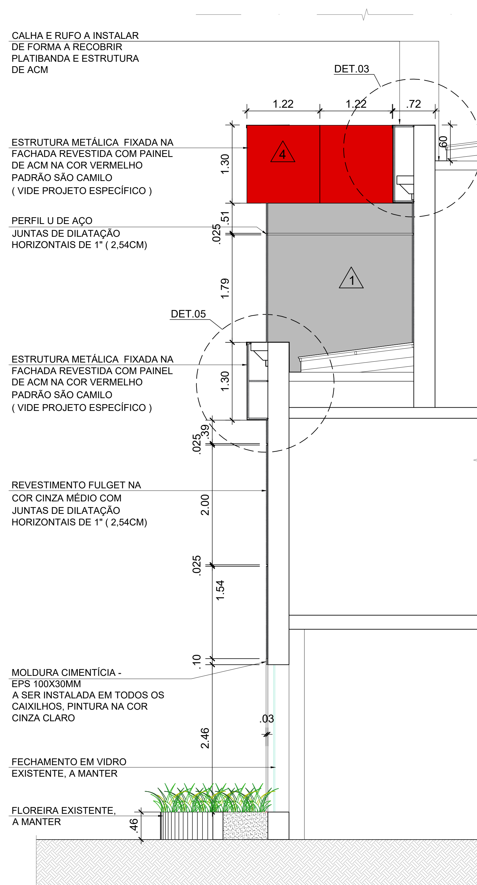
CORTE I-I ESCALA 1:75
