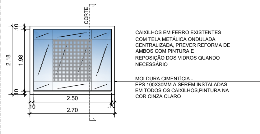
DET. 10 VISTA 3 ( COM TELA METÁLICA ) ESCALA 1:75
