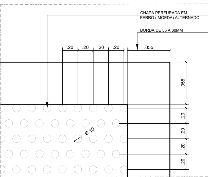
DET. 07 ESCALA 1:25
