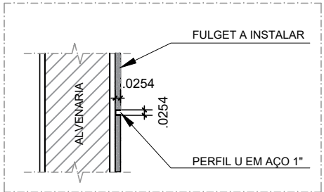
DET. 02 ESCALA: 1:25
