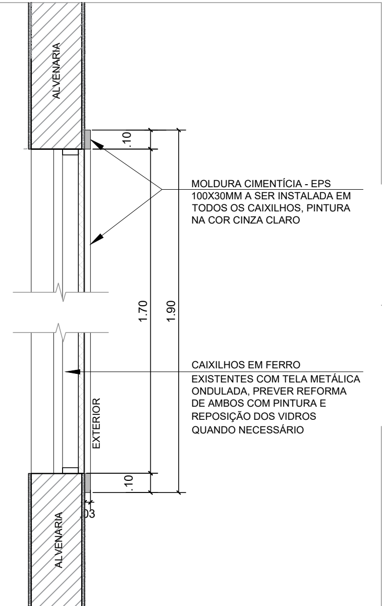
DET. 09 CORTE ( COM TELA METÁLICA ) ESCALA 1:25
