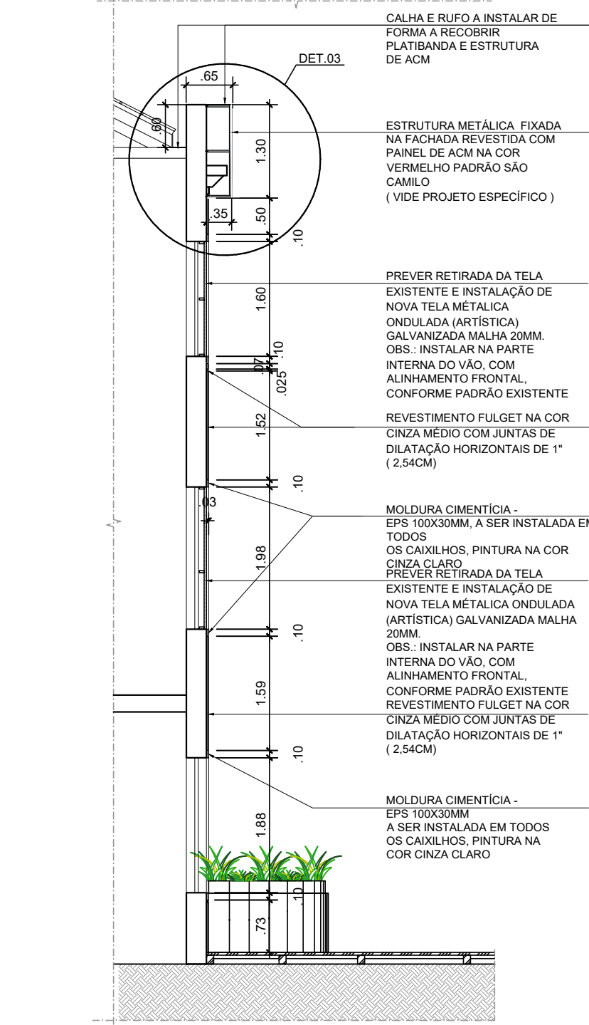
CORTE J-J ESCALA 1:75
