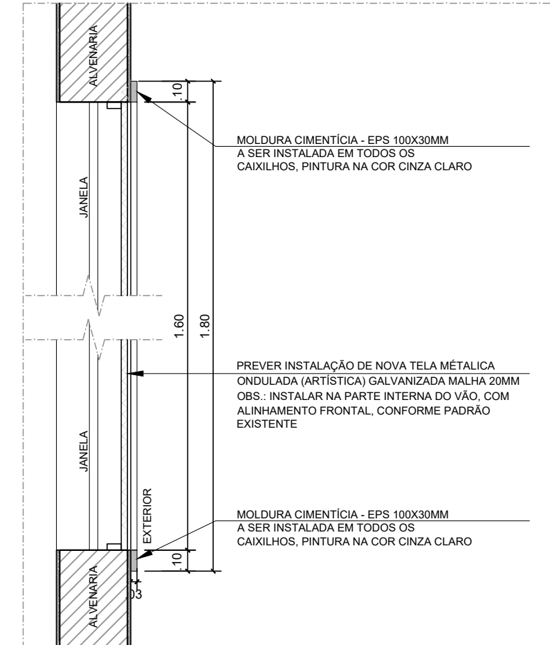
DET. 06- CORTE ( COM TELA METÁLICA ) ESCALA 1:25
