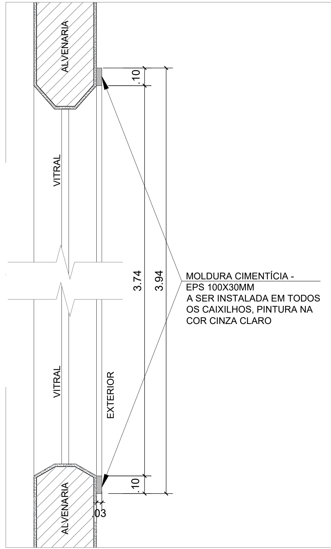
DET. 01 CORTE ( SEM TELA METÁLICA) ESCALA 1:25
