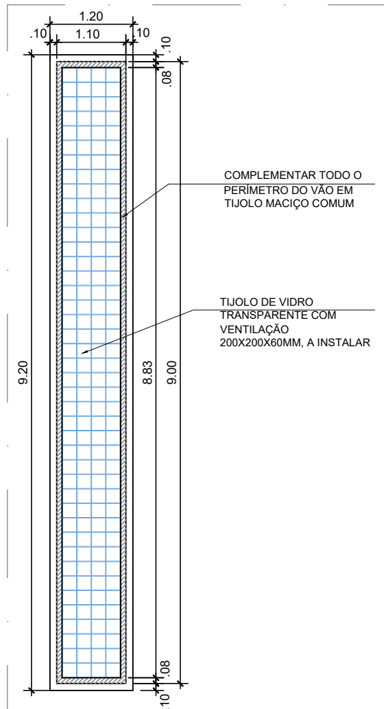
DET. 11 VISTA 2 ESCALA 1:75
