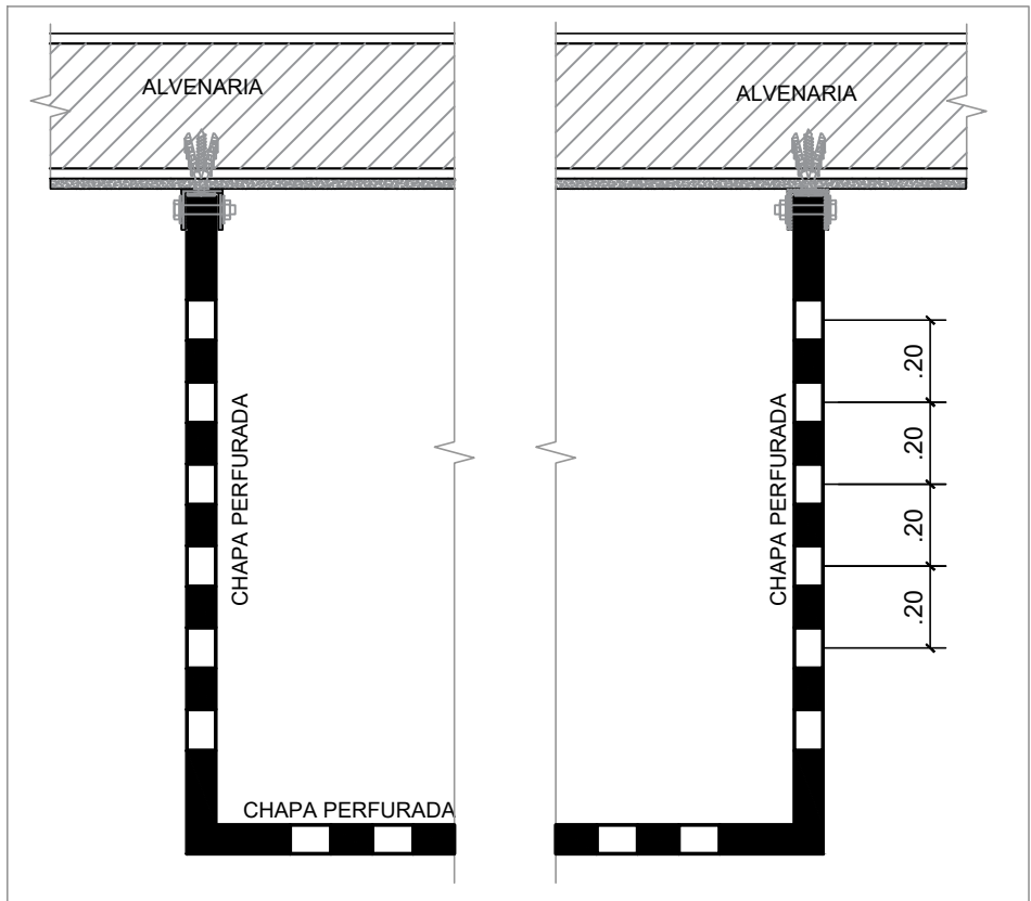
DET. 07- GENÉRICO FIXAÇÃO DA CHAPA PERFORADA ESCALA 1:25
