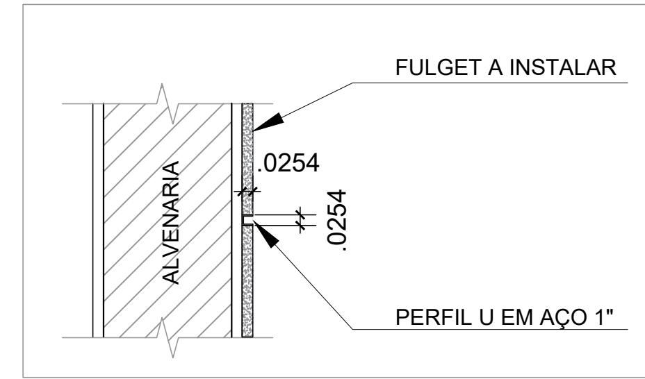
DET. 02 ESCALA 1:25
