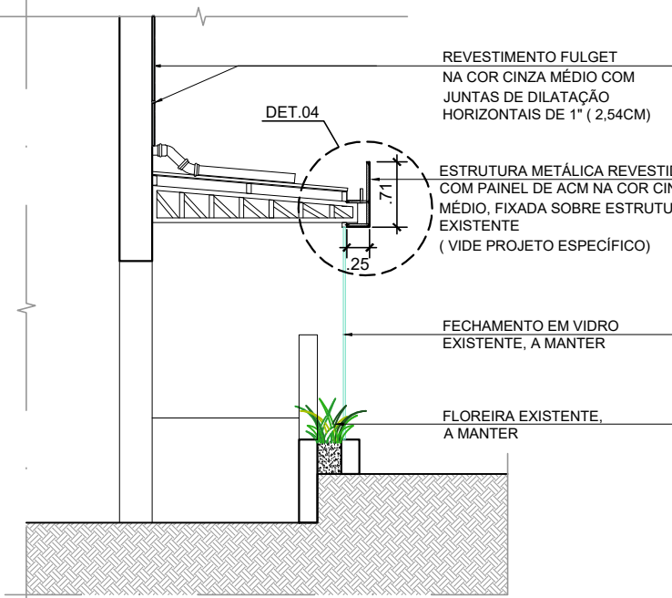
CORTE C-C ESCALA 1:75
