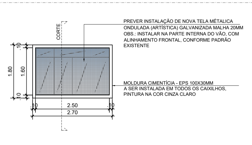
DET. 06- VISTA 5 ( COM TELA METÁLICA ) ESCALA 1:75
