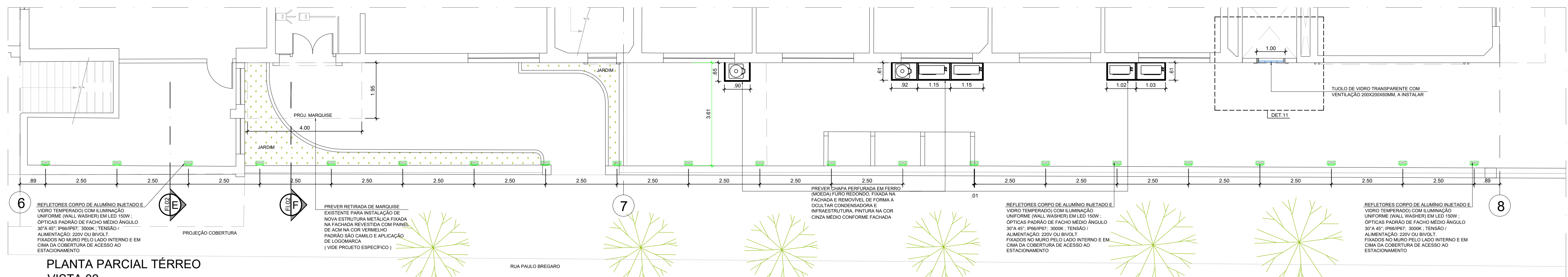
PLANTA PARCIAL TÉRREO VISTA 02 ESCALA: 1:200
