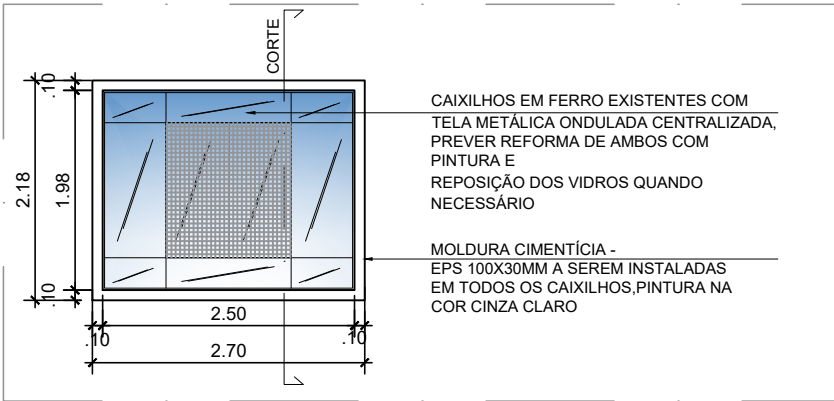
DET. 10 VISTA 3 ( COM TELA METÁLICA ) ESCALA 1:75
