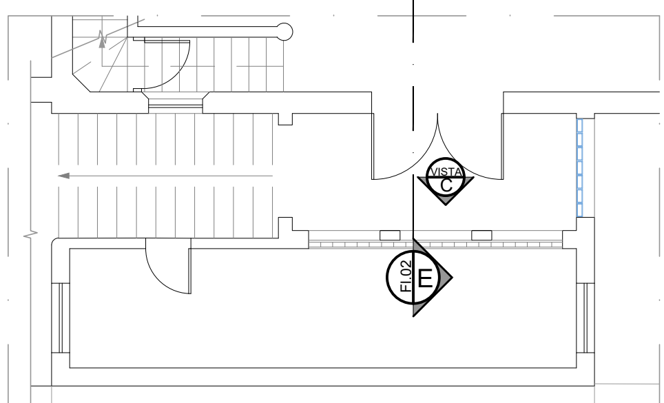
PLANTA PARCIAL 1º ANDAR VISTA 02 ESCALA: 1:200
