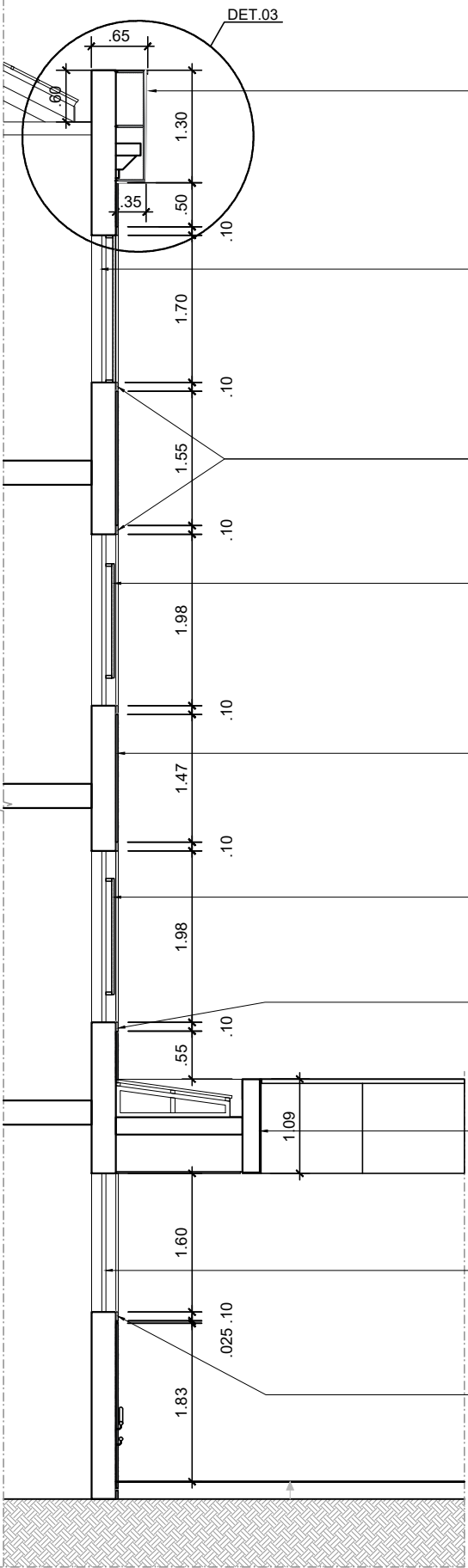
CORTE G - G ESCALA 1:75
