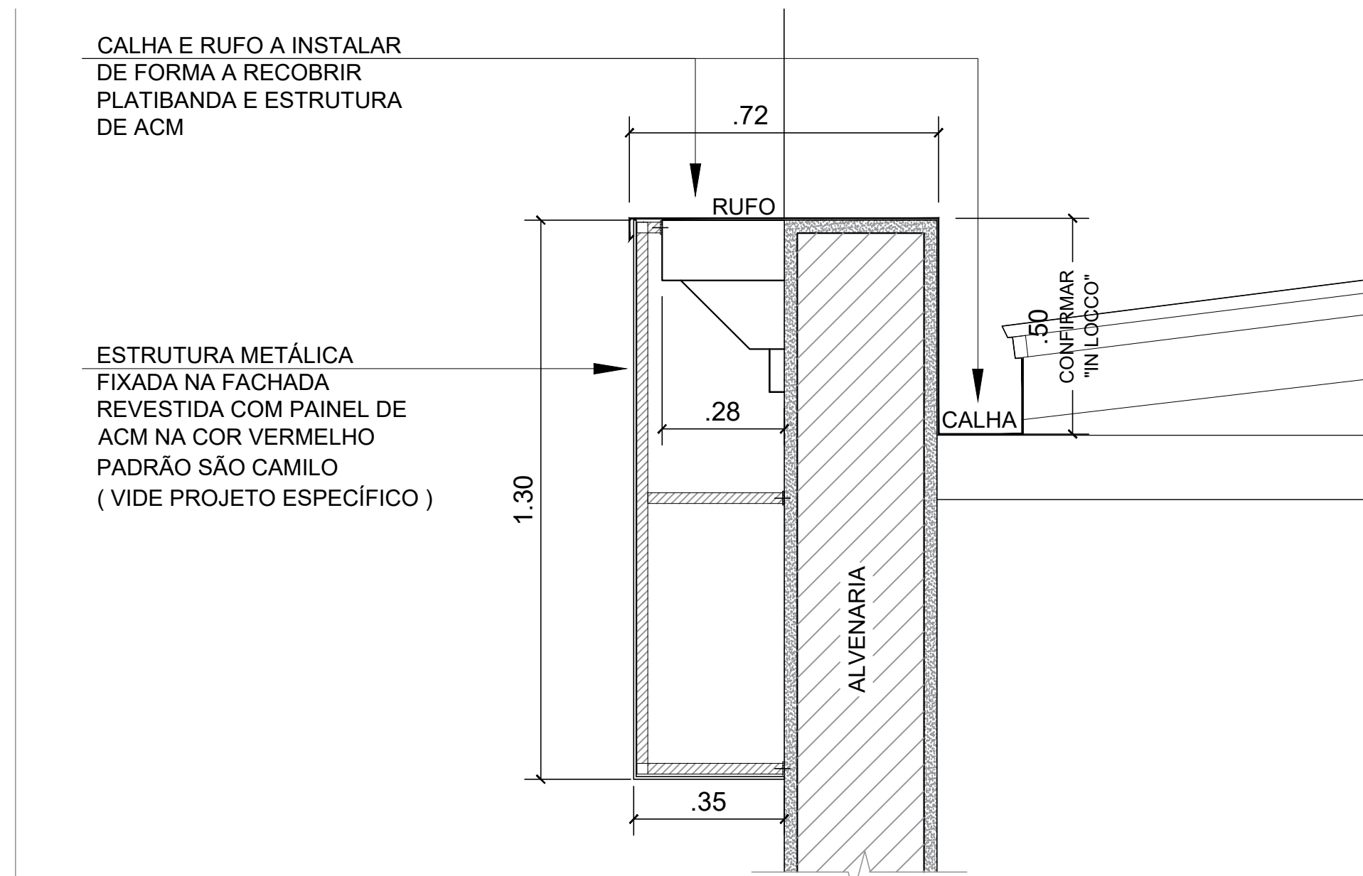
DET. 05 ORIENTATIVO ESCALA 1:25
