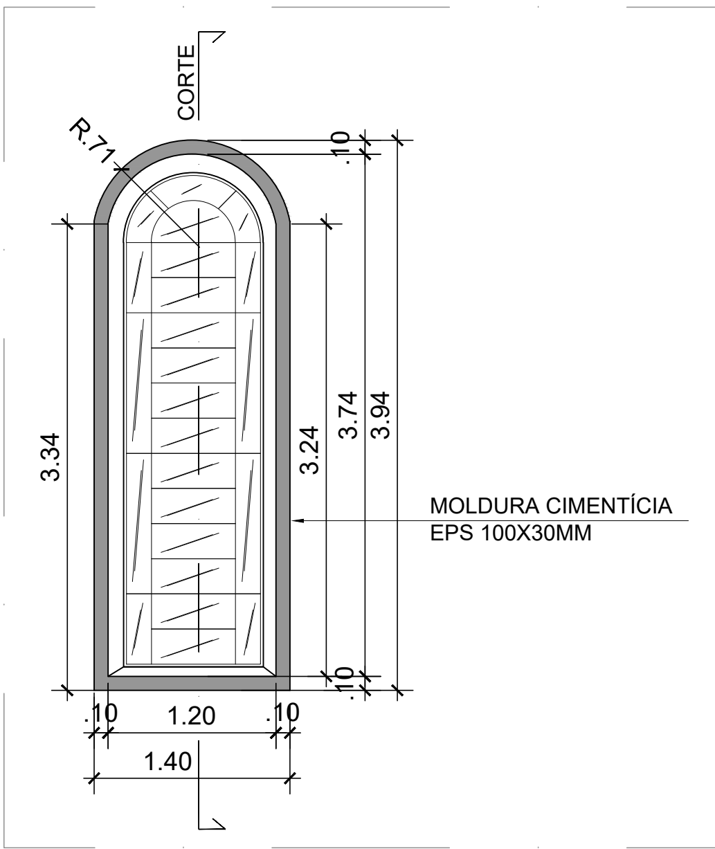
DET. 01 VISTA 4 ( SEM TELA METÁLICA) ESCALA 1:75
