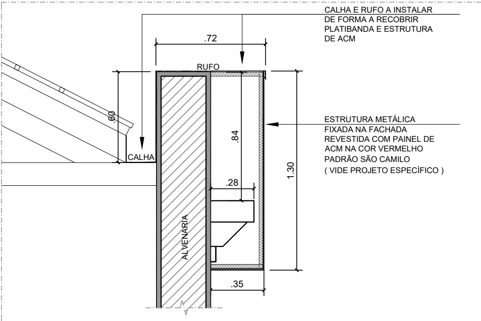
DET. 03-ORIENTATIVO ESCALA 1:25
