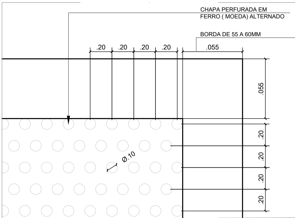
DET. 07 ESCALA 1:25
