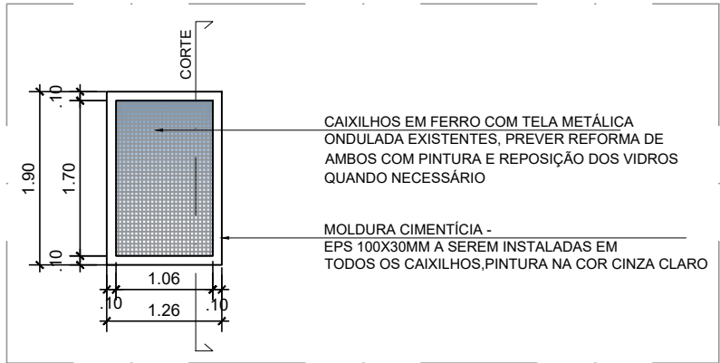
DET. 09 VISTA 1 ( COM TELA METÁLICA ) ESCALA 1:75
