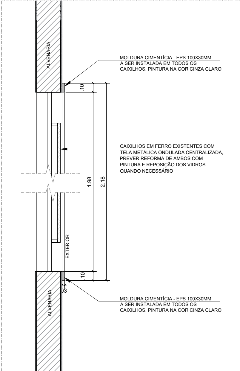
DET. 10 CORTE ( COM TELA METÁLICA ) ESCALA 1:25
