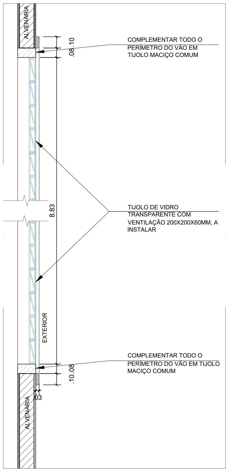
DET. 11- CORTE ( TIJOLO DE VIDRO ) ESCALA 1:25
