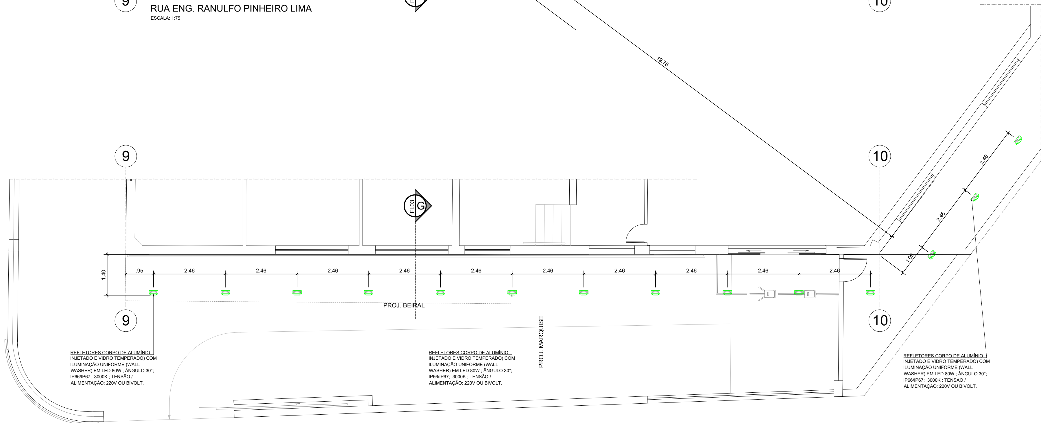
PLANTA PARCIAL VISTA 03 ESCALA: 1:75
