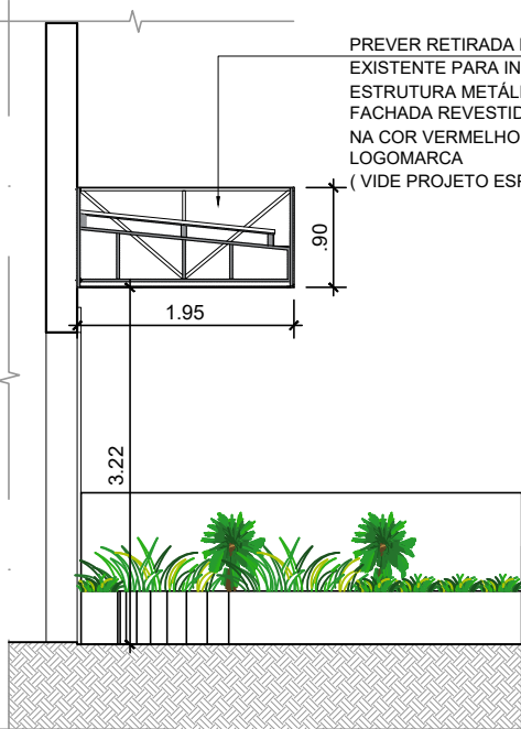
CORTE F-F ESCALA 1:75
