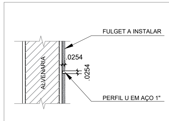
DET. 02 ESCALA 1:25
