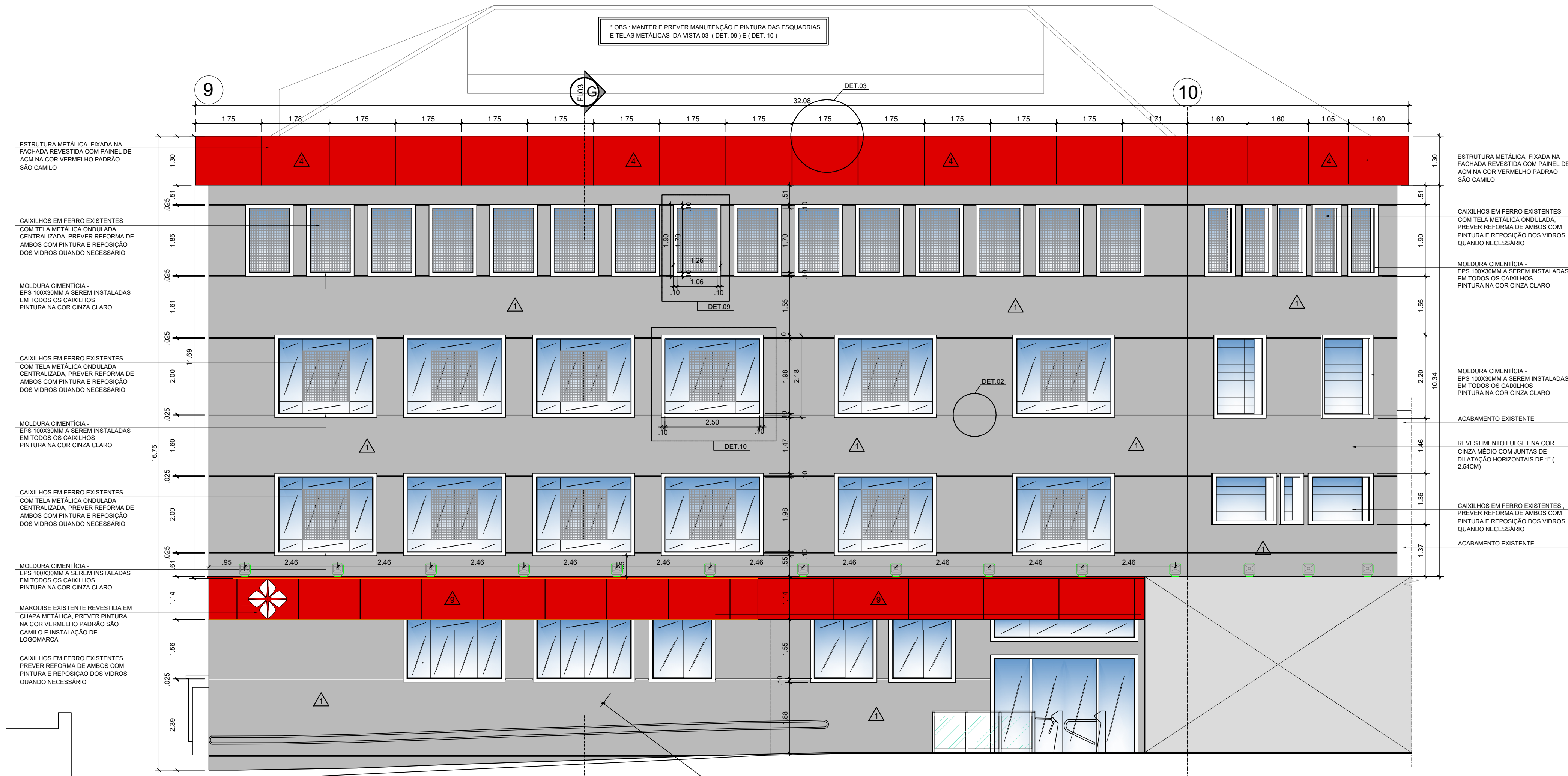
ESCALA: 1:75 VISTA 03 RUA ENG. RANULFO PINHEIRO LIMA ESCALA: 1:75
