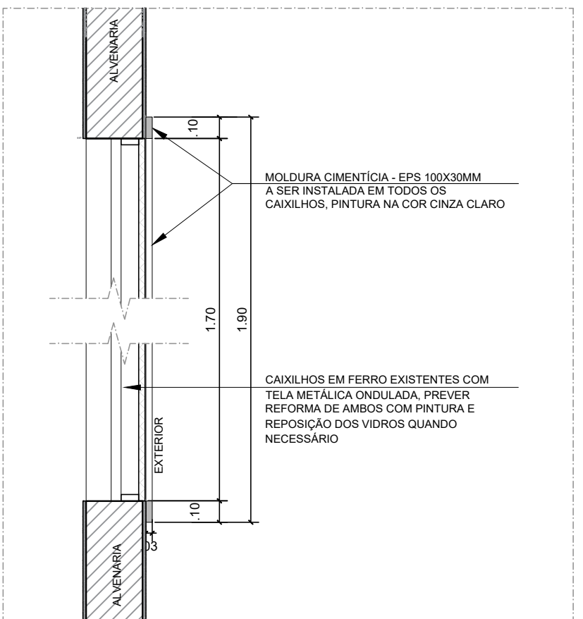
DET. 09- CORTE ( COM TELA METÁLICA ) ESCALA 1:25
