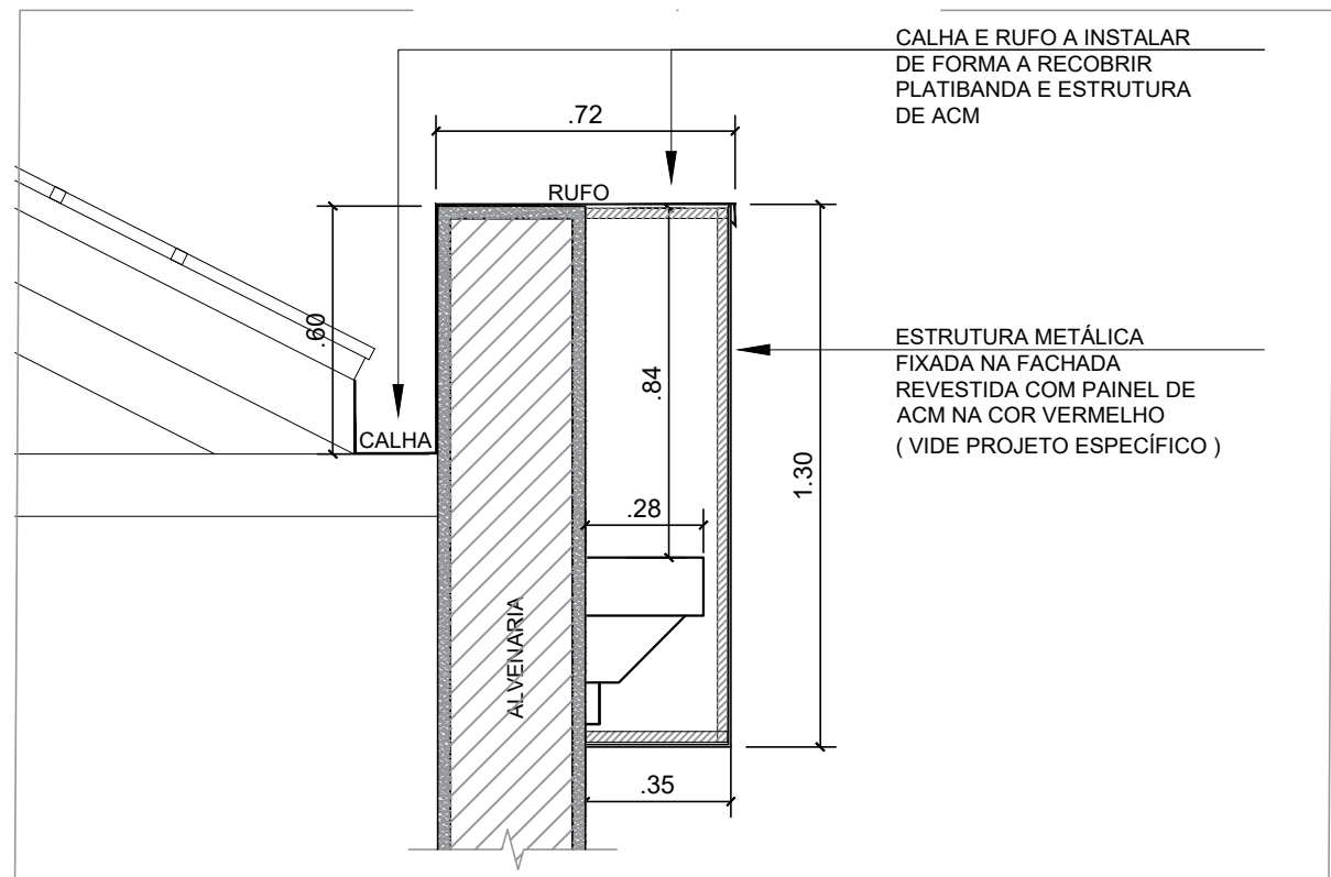
DET. 03 ORIENTATIVO ESCALA 1:25
