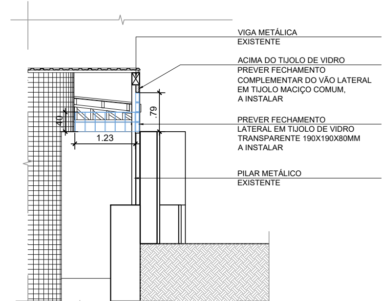
CORTE A-A ESCALA 1:75
