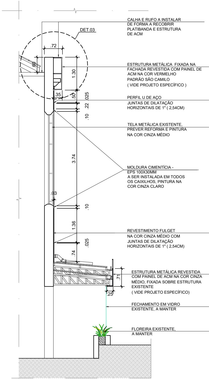
CORTE B-B ESCALA 1:75
