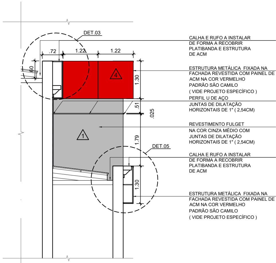
CORTE D-D ESCALA 1:75
