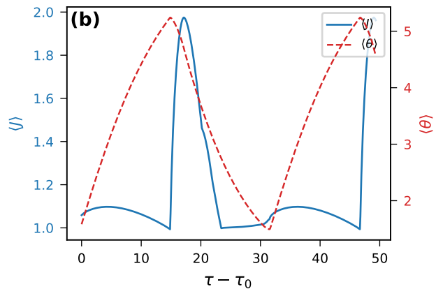
Regime I: S_\chi = 0.7 , Da = 4.0 (volume pulse)
