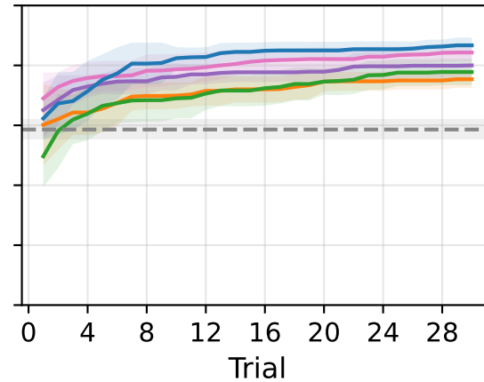
MultiHop-RAG
