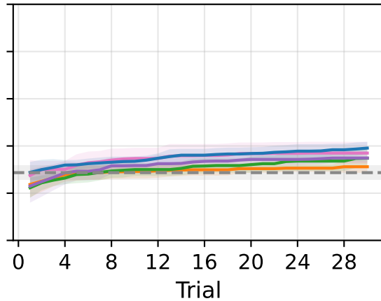
MuSiQue
