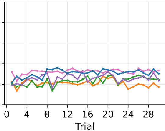
MuSiQue
