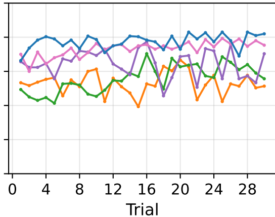
MultiHop-RAG
