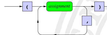
arglist
