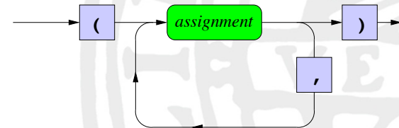
arglist
