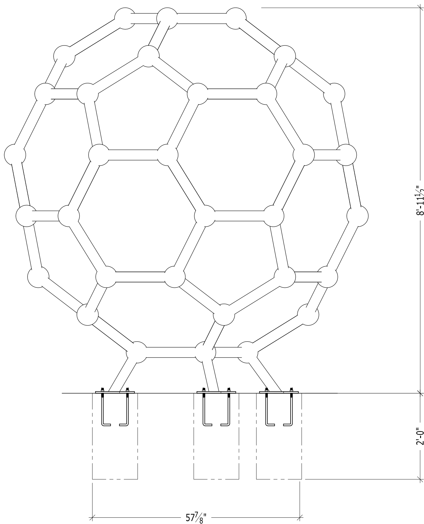
A ELEVATION - SCALE: 3/4" = 1'-0"
